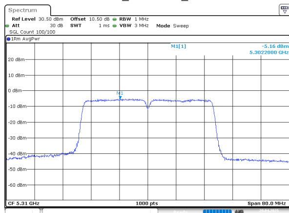
802.11n40_5310MHz_Chain 0
