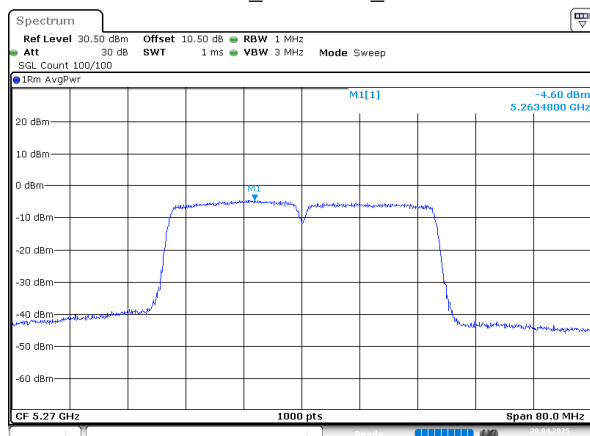
802.11n40_5270MHz_Chain 0
