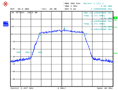
802.11n20_2437MHz_Chain 0
