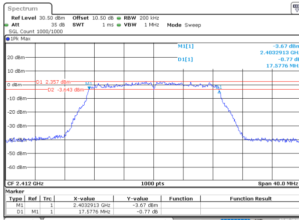
802.11n20_2412MHz_Chain 0
