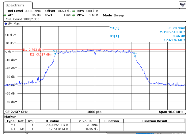
802.11n20_2437MHz_Chain 0
