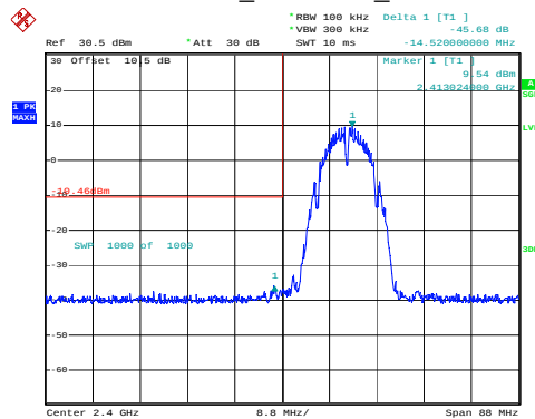
802.11b_2412MHz_Chain 1
