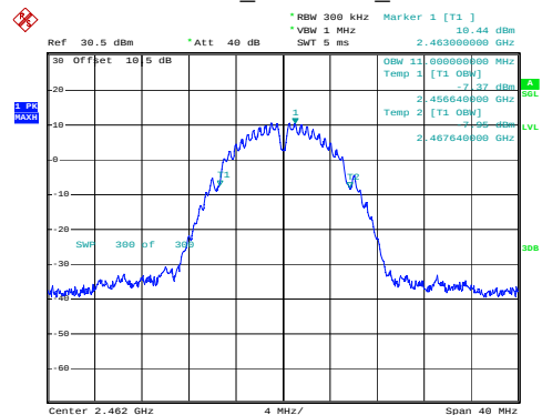
802.11b_2462MHz_Chain 1
