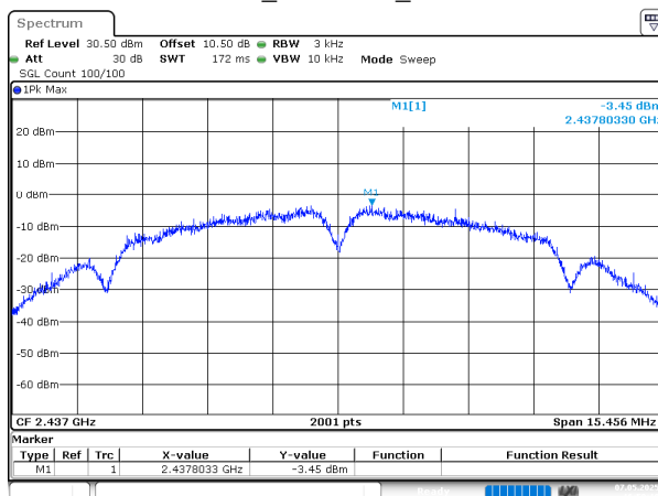
802.11b_2437MHz_Chain 1
