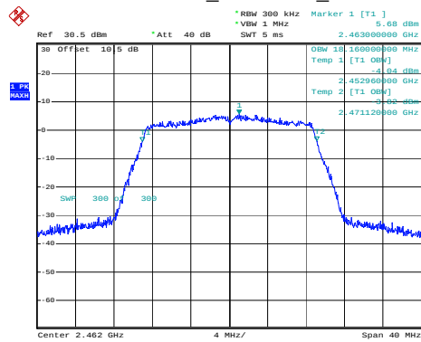
802.11n20_2462MHz_Chain 0
