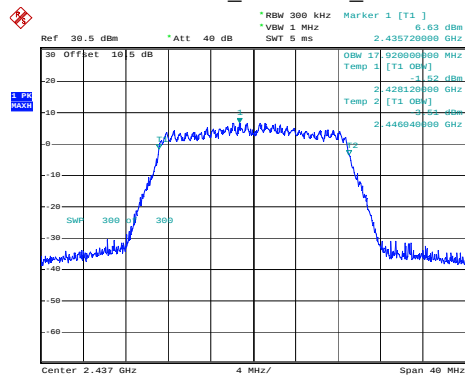
802.11n20_2437MHz_Chain 1
