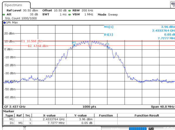
802.11b_2437MHz_Chain 1
