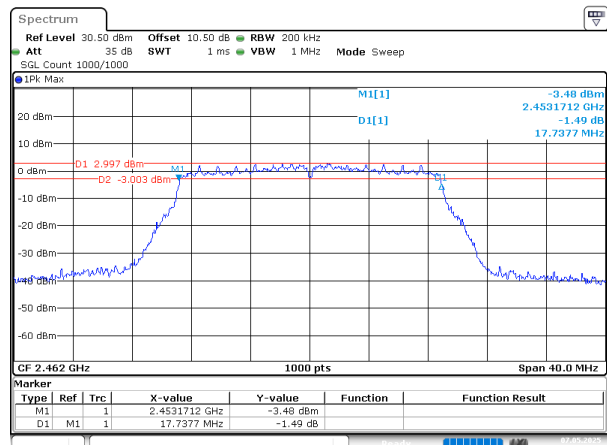
802.11n20_2462MHz_Chain 1
