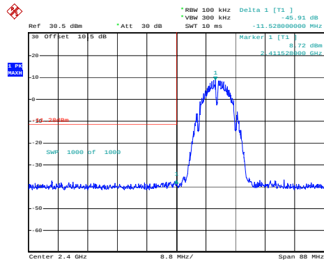
802.11b_2412MHz_Chain 0
