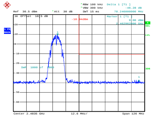
802.11b_2462MHz_Chain 0
