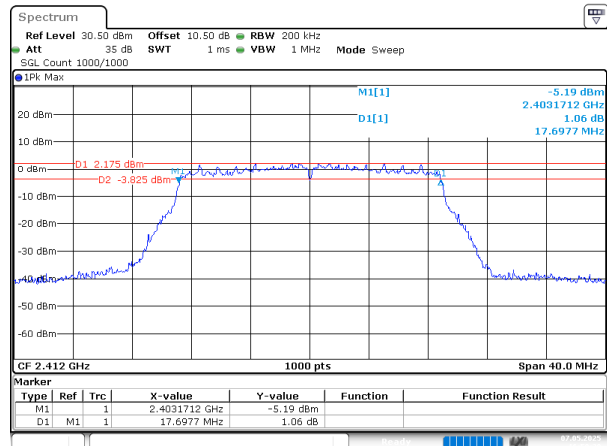
802.11n20_2412MHz_Chain 1
