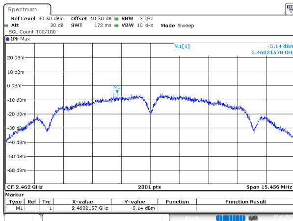
802.11b_2462MHz_Chain 0
