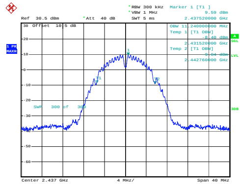
802.11b_2437MHz_Chain 0
