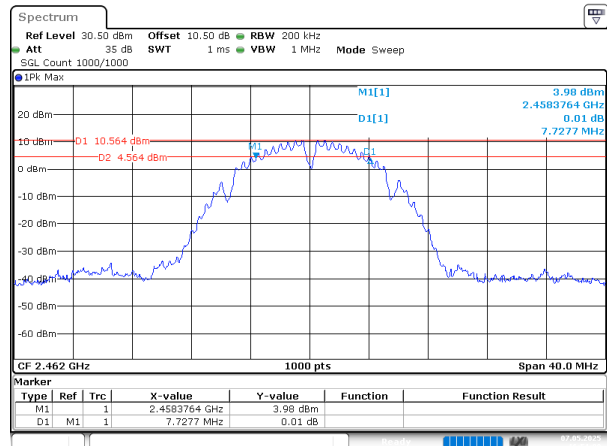
802.11b_2462MHz_Chain 1
