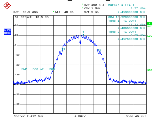
802.11b_2412MHz_Chain 1
