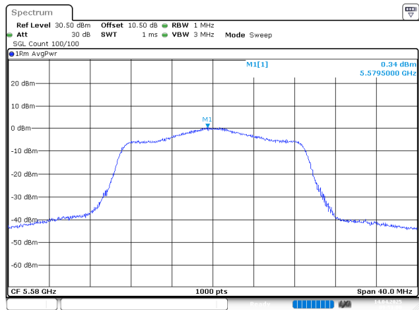
802.11n20_5580MHz_Chain 1
