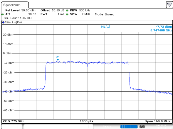
802.11ax80_5775MHz_Chain 1
