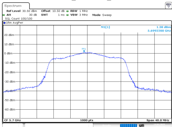
802.11n20_5700MHz_Chain 0
