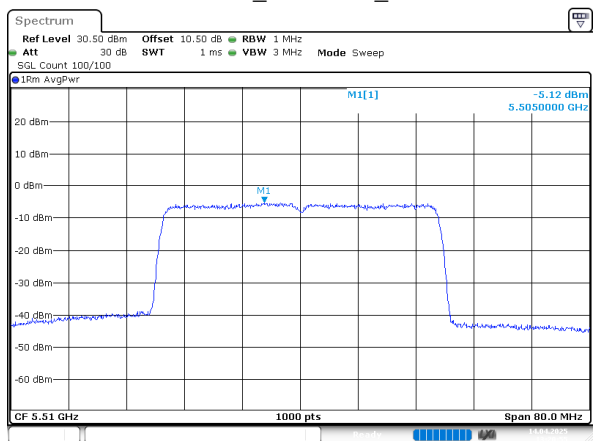
802.11ax40_5510MHz_Chain 0
