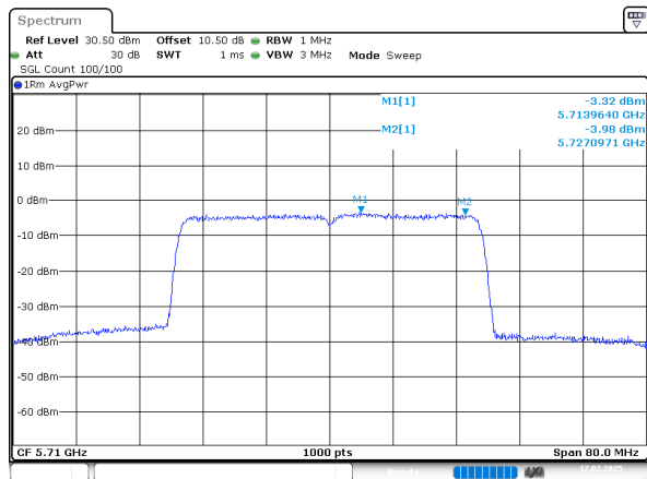
802.11ax40_5710MHz_Chain 1
