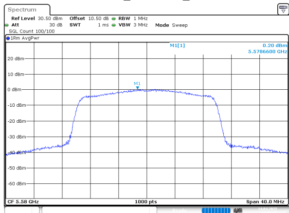
802.11ax20_5580MHz_Chain 1
