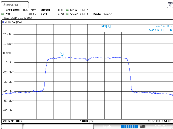
802.11ax40_5310MHz_Chain 0
