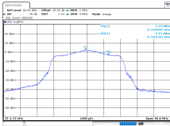
802.11a_5720MHz_Chain 1
