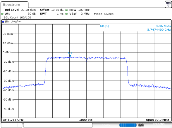
802.11ax40_5755MHz_Chain 1
