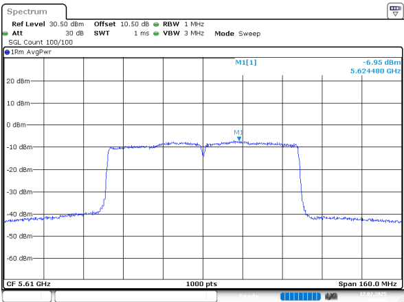
802.11ac80_5610MHz_Chain 1
