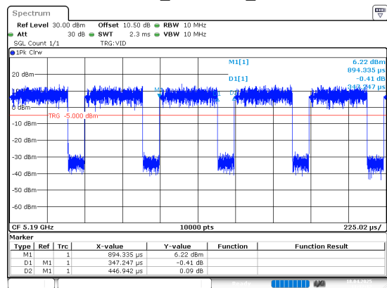
802.11n40_5190MHz_Chain 0
