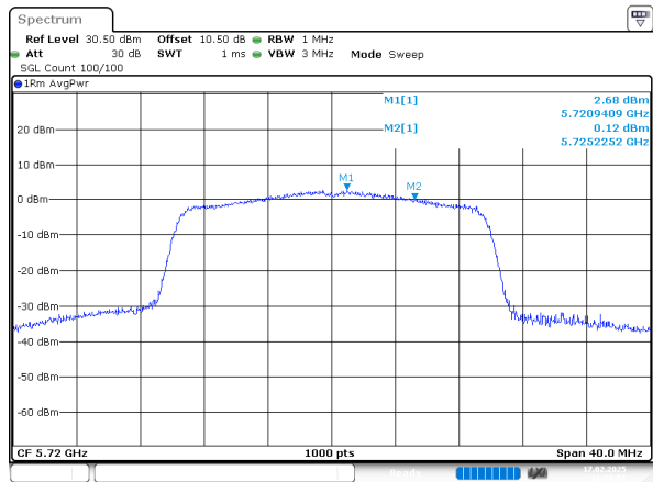
802.11ax20_5720MHz_Chain 1
