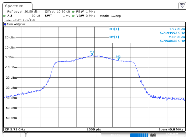
802.11n20_5720MHz_Chain 1
