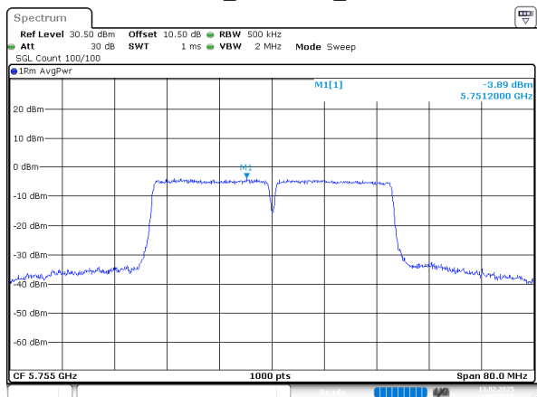
802.11n40_5755MHz_Chain 0
