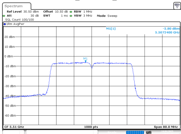
802.11n40_5510MHz_Chain 0
