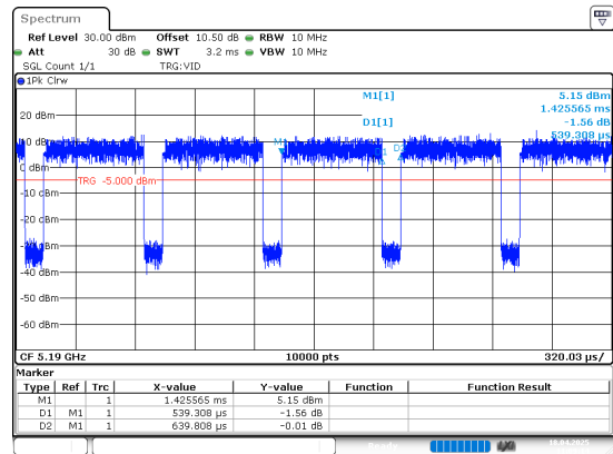
802.11ax40_5190MHz_Chain 0
