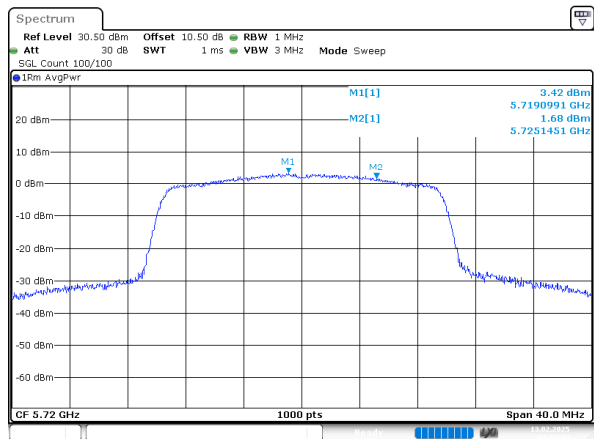
802.11ax20_5720MHz_Chain 0
