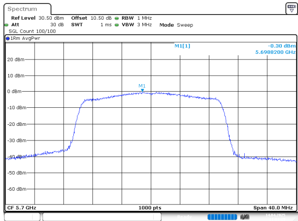
802.11ax20_5700MHz_Chain 1
