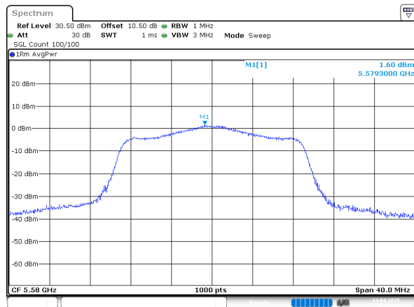
802.11n20_5580MHz_Chain 0
