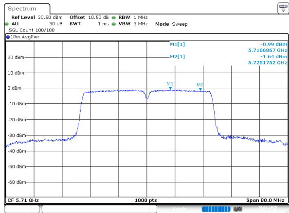
802.11n40_5710MHz_Chain 0
