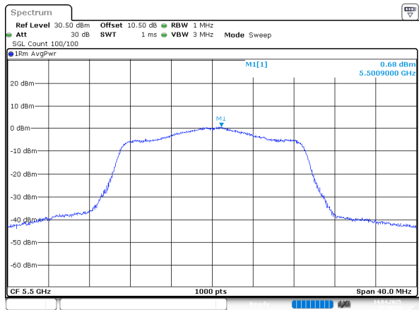
802.11n20_5500MHz_Chain 1
