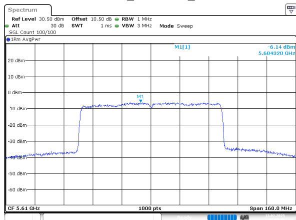
802.11ax80_5610MHz_Chain 0
