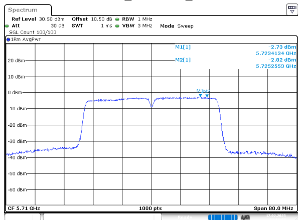
802.11n40_5710MHz_Chain 1
