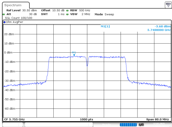
802.11n40_5755MHz_Chain 1
