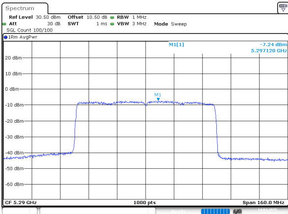
802.11ax80_5290MHz_Chain 1
