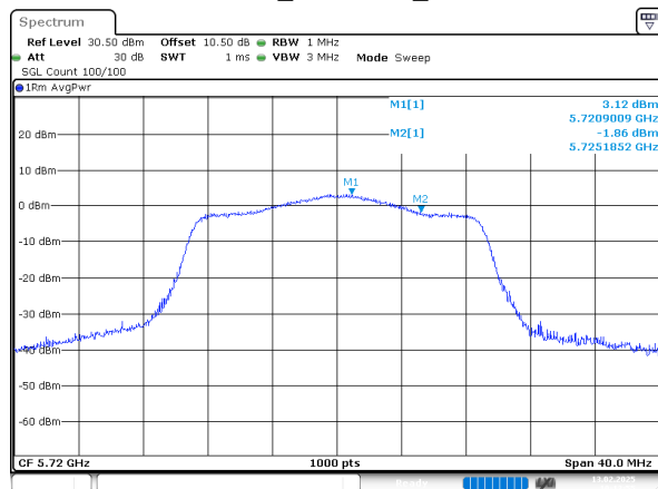
802.11n20_5720MHz_Chain 0
