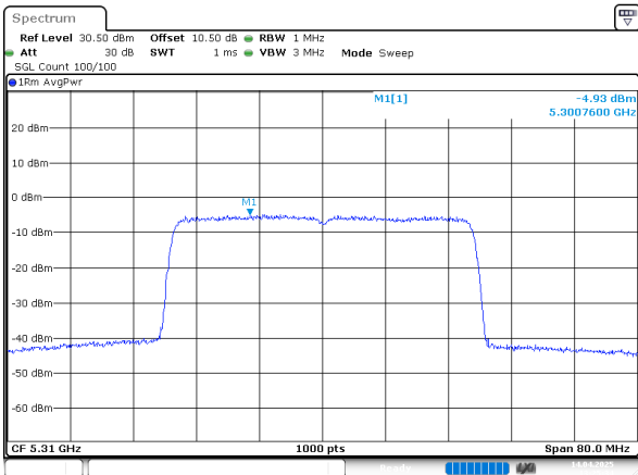
802.11ax40_5310MHz_Chain 1
