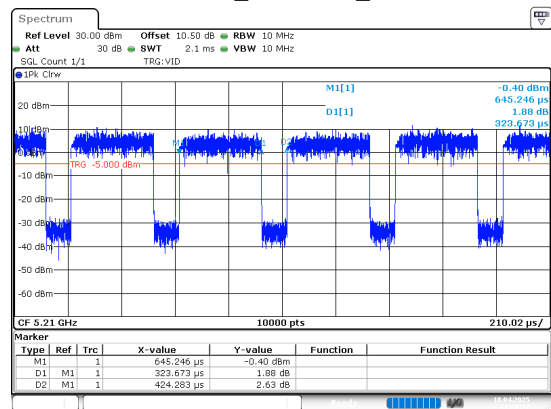
802.11ac80_5210MHz_Chain 0
