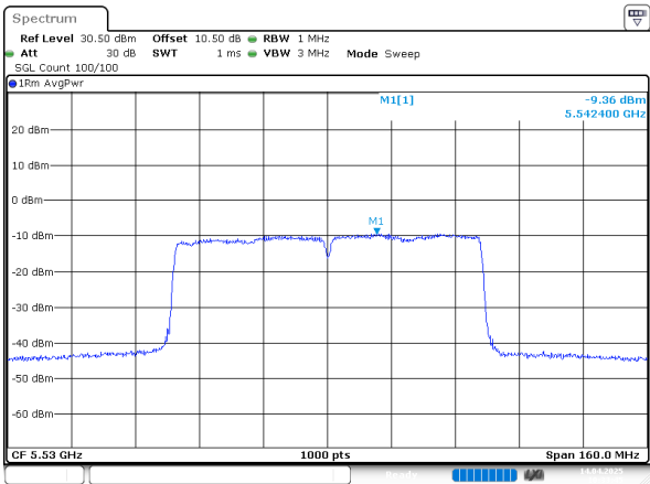
802.11ac80_5530MHz_Chain 1
