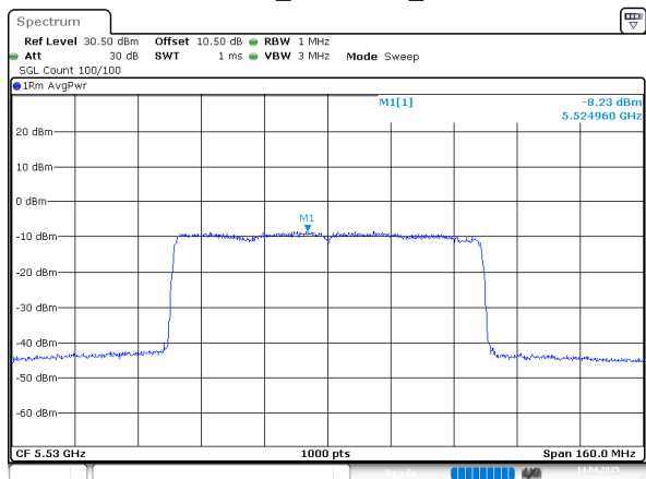
802.11ax80_5530MHz_Chain 0
