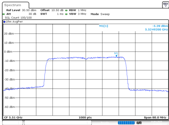
802.11ax40_5510MHz_Chain 1
