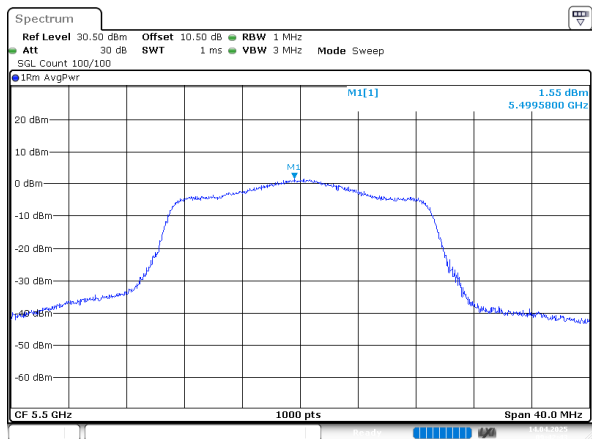
802.11n20_5500MHz_Chain 0
