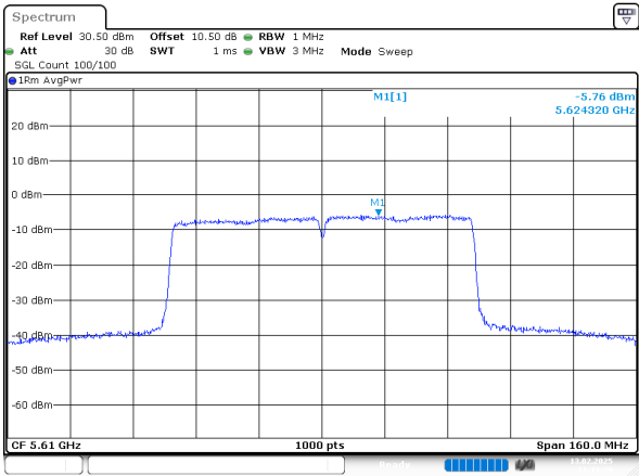
802.11ac80_5610MHz_Chain 0
