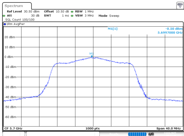
802.11n20_5700MHz_Chain 1
