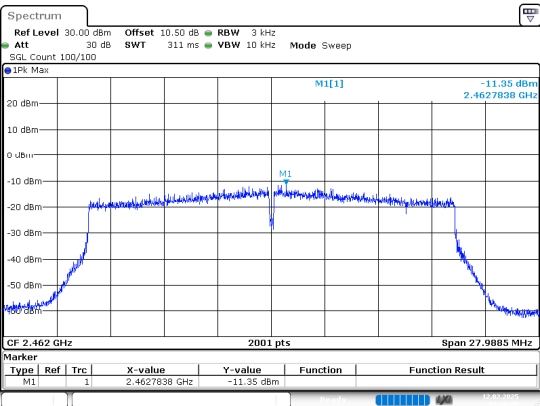
802.11ax20_2462MHz_Chain 0
