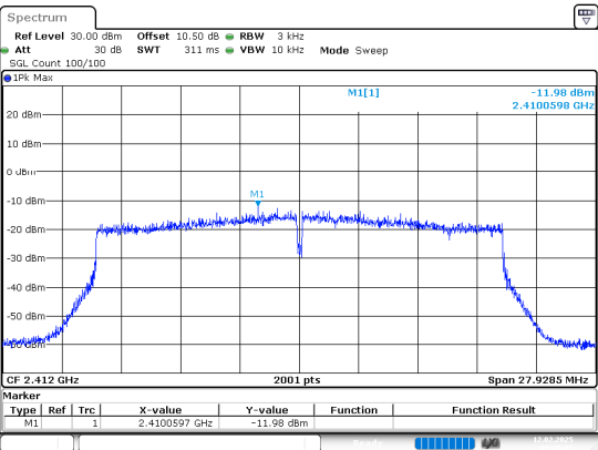
802.11ax20_2412MHz_Chain 1
