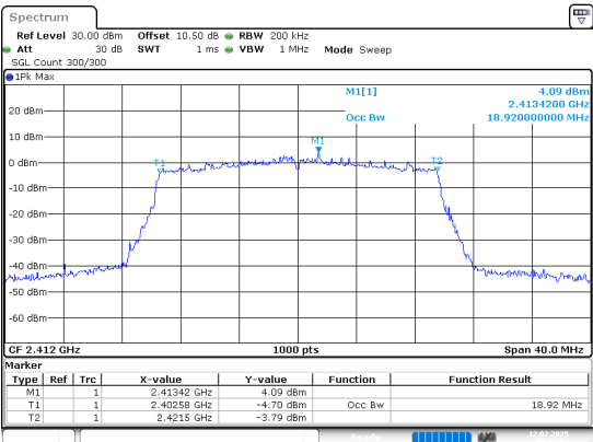
802.11ax20_2412MHz_Chain 1
