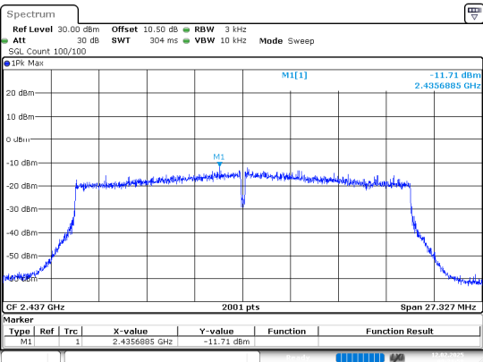
802.11ax20_2437MHz_Chain 1
