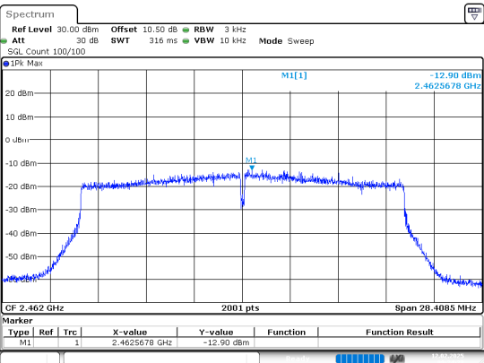
802.11ax20_2462MHz_Chain 1
