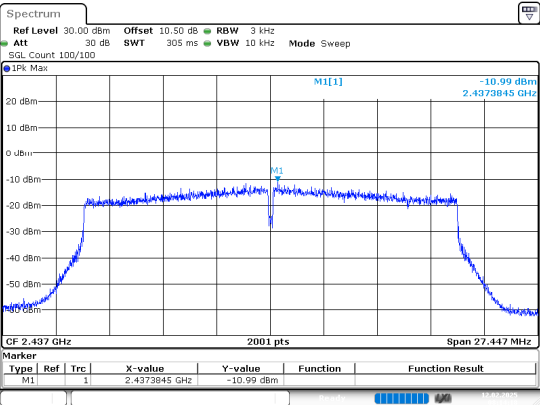
802.11ax20_2437MHz_Chain 0
