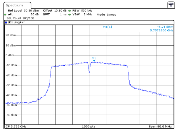
802.11ac40_5755MHz
