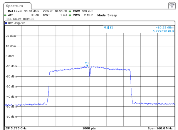
802.11ac80_5775MHz
