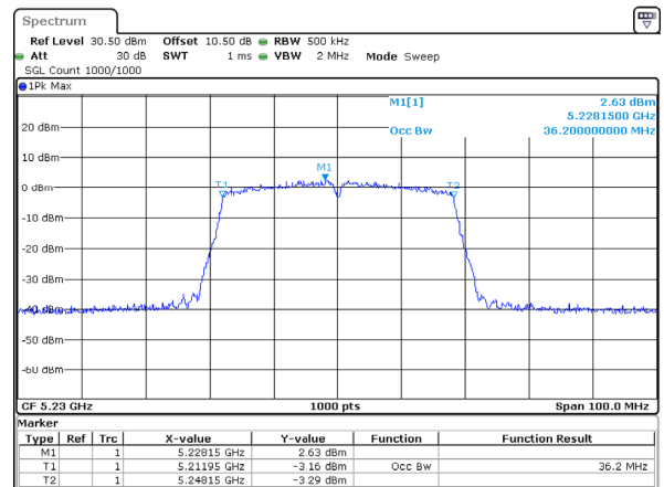
802.11ac40_5230MHz
