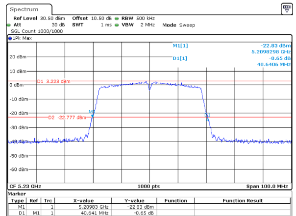
802.11ac40_5230MHz
