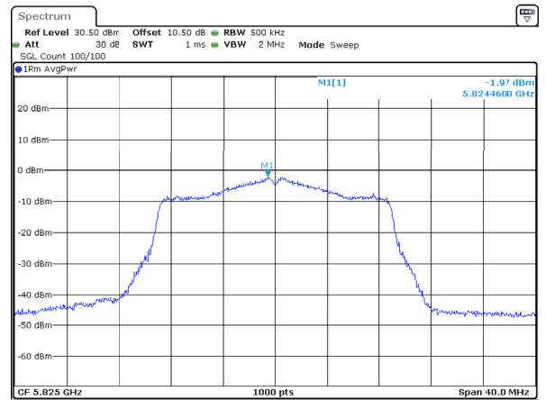
802.11ac20_5825MHz_Chain 2
