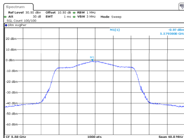
802.11ac20_5580MHz_Chain 1
