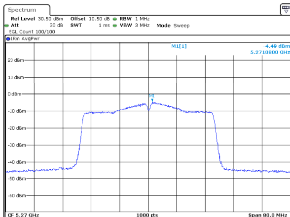
802.11ac40_5270MHz_Chain 2
