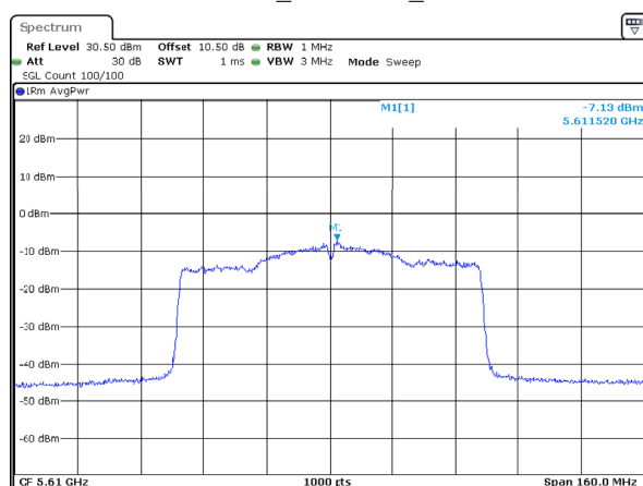
802.11ac80_5610MHz_Chain 2
