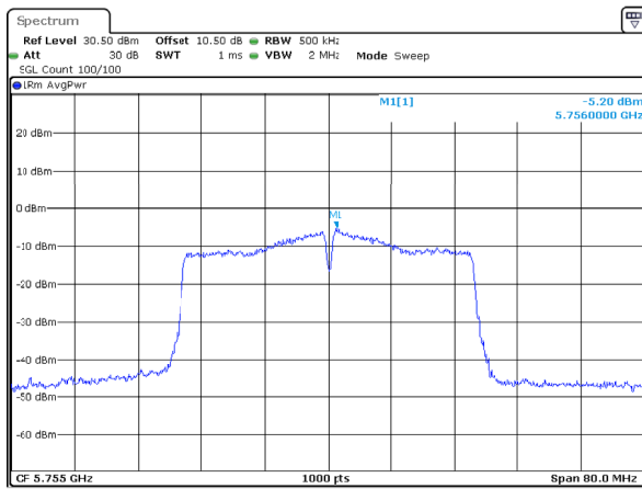
802.11ac40_5755MHz_Chain 2
