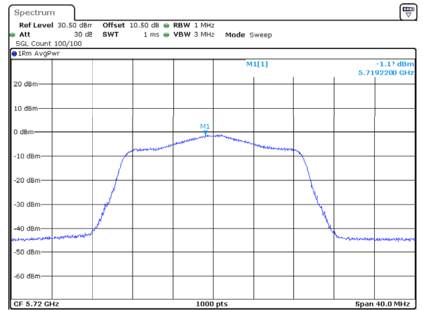
802.11ac20_5720MHz_Chain 2
