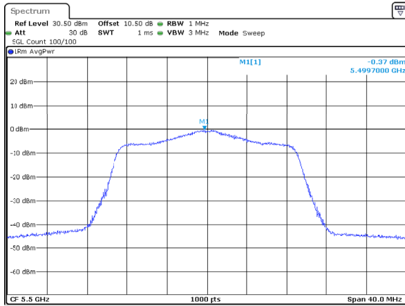
802.11ac20_5500MHz_Chain 2
