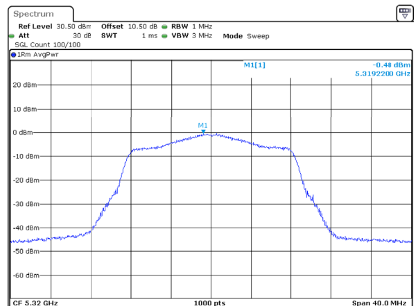
802.11a_5320MHz_Chain 2
