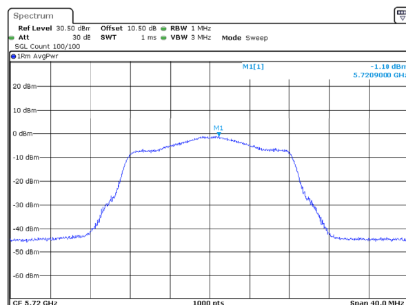
802.11a_5720MHz_Chain 2
