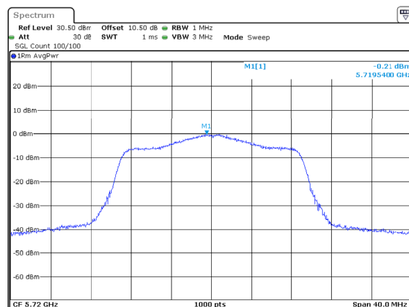
802.11ac20_5720MHz_Chain 1
