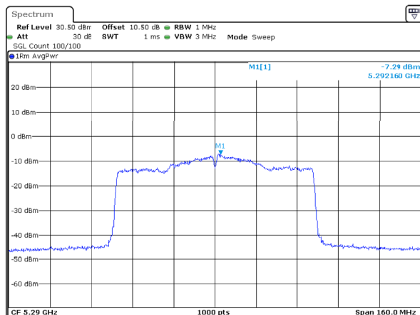
802.11ac80_5290MHz_Chain 2
