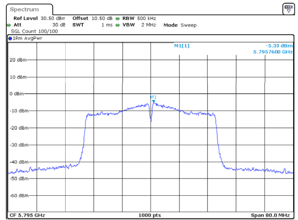
802.11ac40_5795MHz_Chain 2
