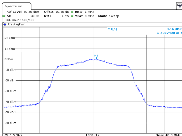
802.11a_5500MHz_Chain 2
