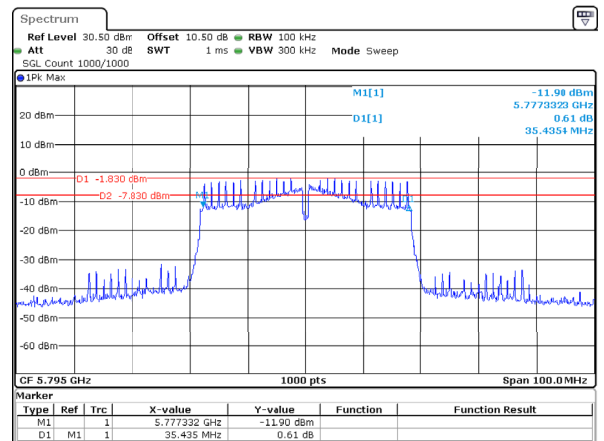
802.11ac40_5795MHz_Chain 2
