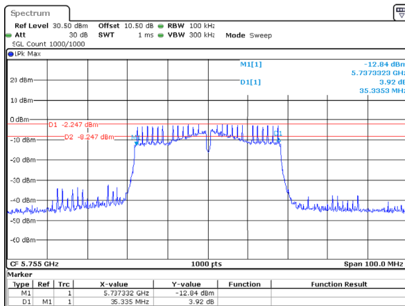
802.11ac40_5755MHz_Chain 2
