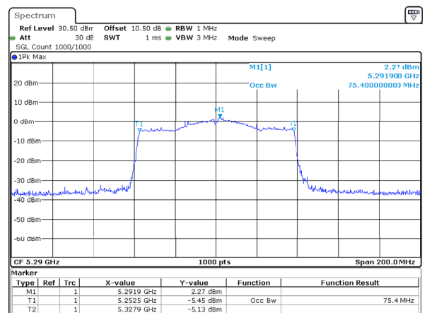
802.11ac80_5290MHz_Chain 2
