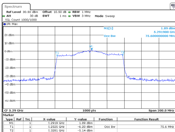
802.11ac80_5290MHz_Chain 1
