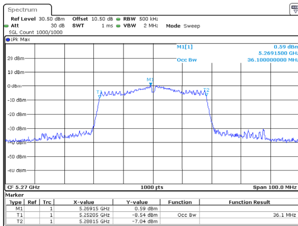
802.11ac40_5270MHz_Chain 1
