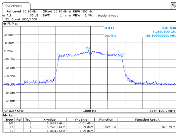
802.11ac40_5270MHz_Chain 2
