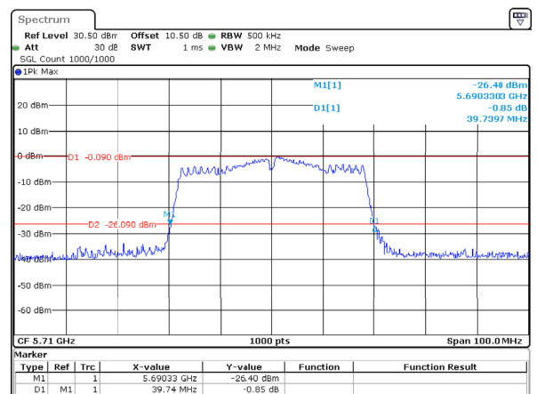
802.11ac40_5710MHz_Chain 2
