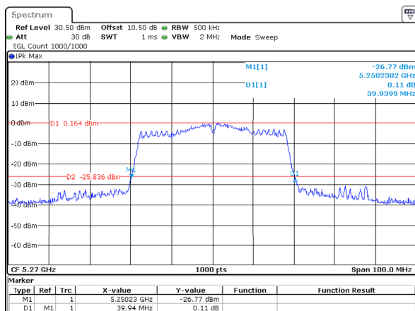
802.11ac40_5270MHz_Chain 1
