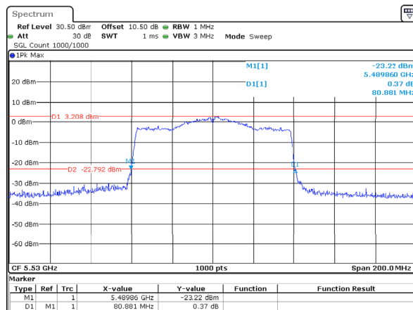
802.11ac80_5530MHz_Chain 2
