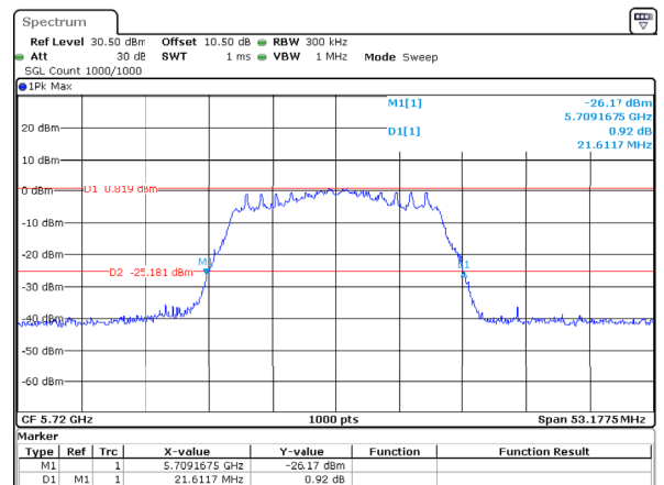
802.11ac20_5720MHz_Chain 2
