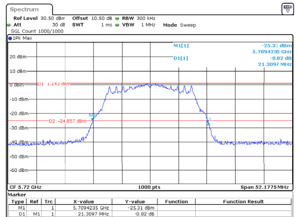
802.11a_5720MHz_Chain 2
