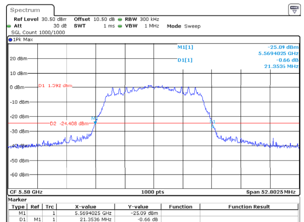
802.11ac20_5580MHz_Chain 1
