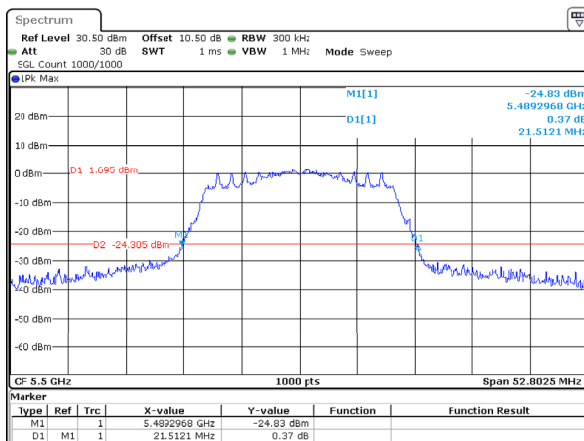
802.11ac20_5500MHz_Chain 1
