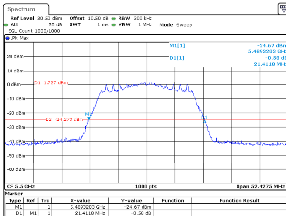
802.11ac20_5500MHz_Chain 2
