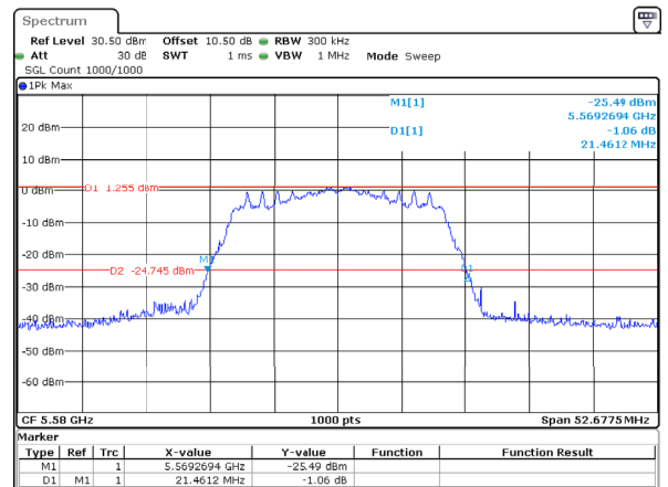
802.11ac20_5580MHz_Chain 2
