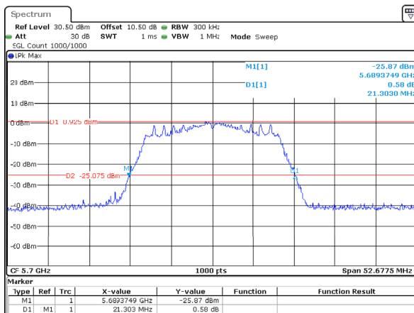
802.11ac20_5700MHz_Chain 2
