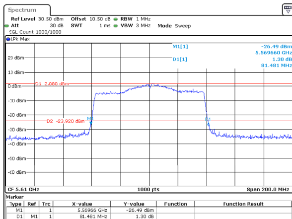
802.11ac80_5610MHz_Chain 2
