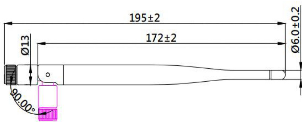
天线尺寸/ANT Size(Unit:mm)
