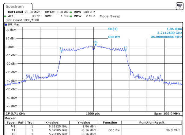
802.11ac40_5710MHz
