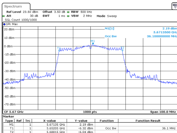
802.11ac40_5670MHz
