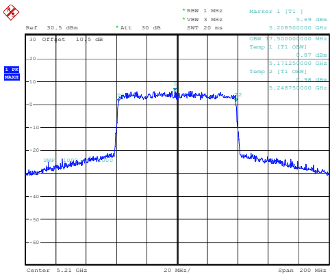
802.11ax80_5210MHz_RU_Full
