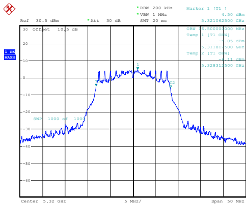
802.11a_5320MHz
