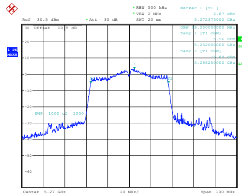
802.11ac40_5270MHz
