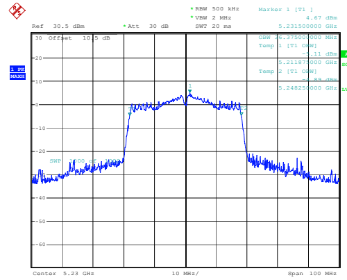
802.11ac40_5230MHz
