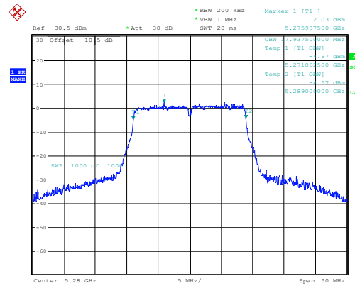
802.11ac20_5280MHz
