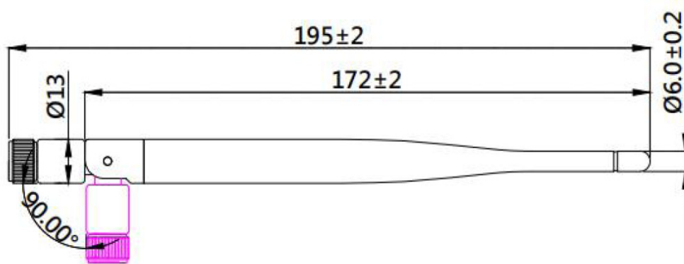
天线尺寸/ANT Size(Unit:mm)
