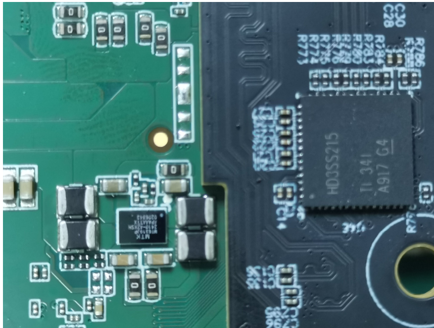
Module YL7981
