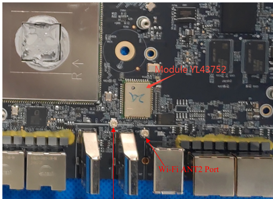
BLE ANT/Wi-Fi ANT1 Port
