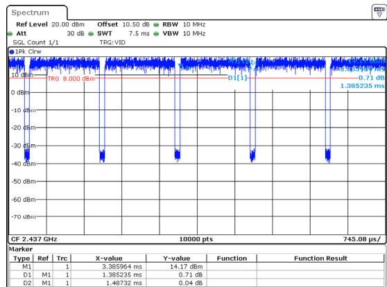
802.11g_2437MHz
