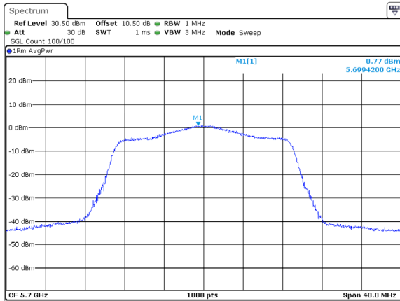
802.11ac20_5700MHz_Chain 2
