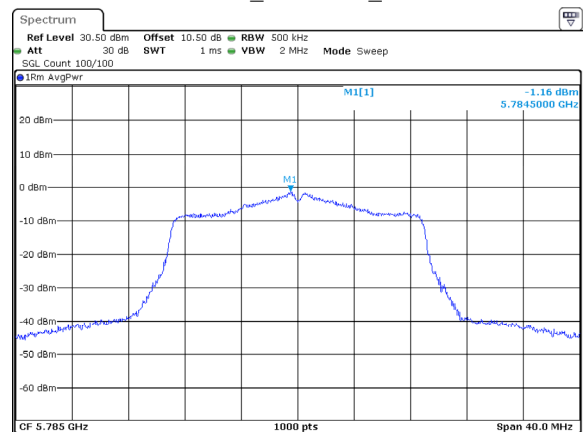
802.11ac20_5785MHz_Chain 1
