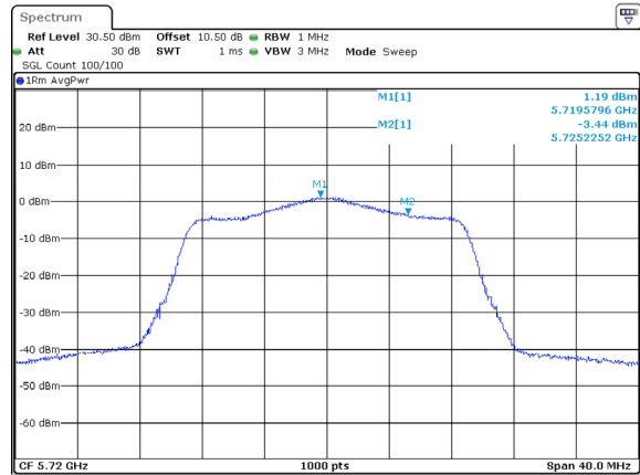
802.11ac20_5720MHz_Chain 2
