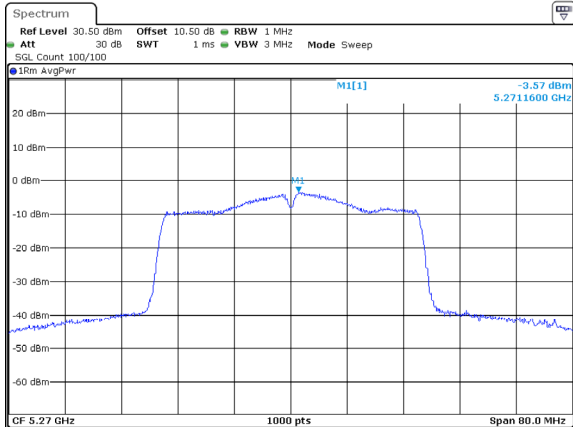
802.11ac40_5270MHz_Chain 1
