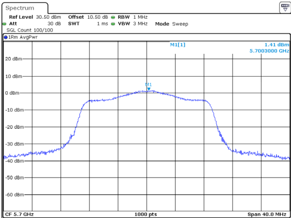
802.11ac20_5700MHz_Chain 1
