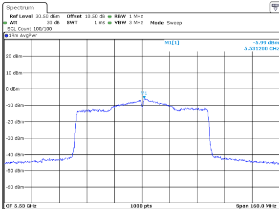
802.11ac80_5530MHz_Chain 1
