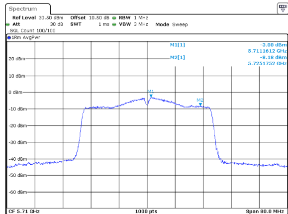
802.11ac40_5710MHz_Chain 2
