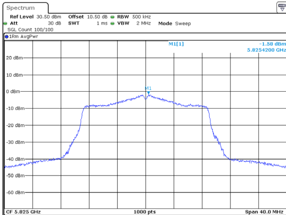
802.11ac20_5825MHz_Chain 1
