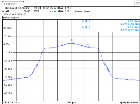
802.11a_5720MHz_Chain 2
