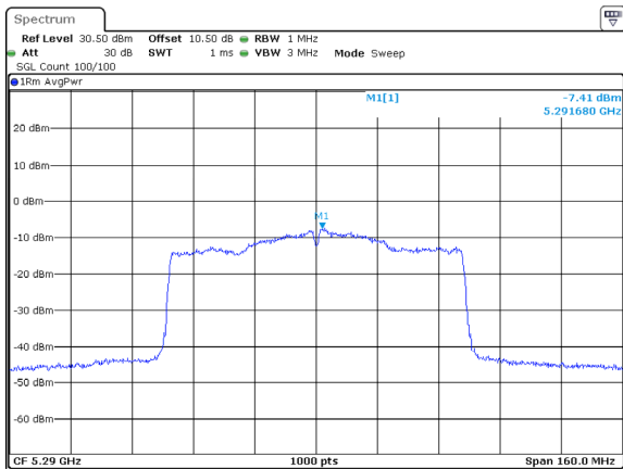
802.11ac80_5290MHz_Chain 1
