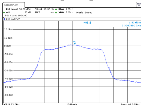
802.11ac20_5320MHz_Chain 2
