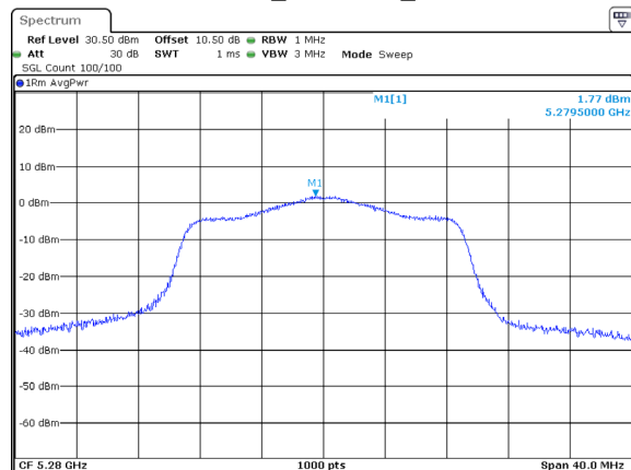
802.11ac20_5280MHz_Chain 1
