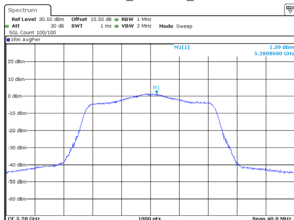
802.11ac20_5280MHz_Chain 2
