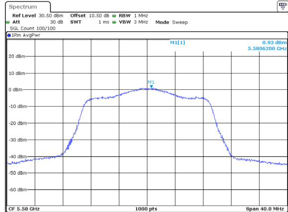
802.11ac20_5580MHz_Chain 2
