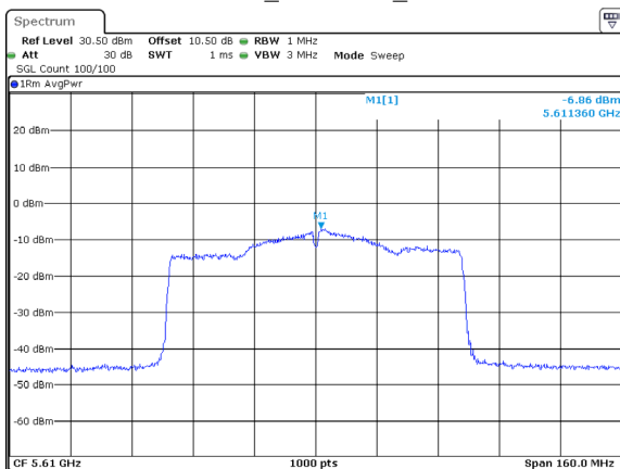
802.11ac80_5610MHz_Chain 2
