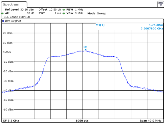
802.11ac20_5500MHz_Chain 1
