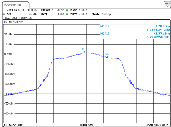
802.11a_5720MHz_Chain 1
