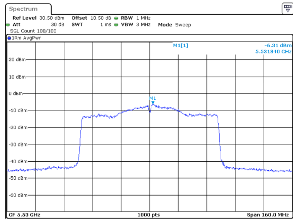
802.11ac80_5530MHz_Chain 2
