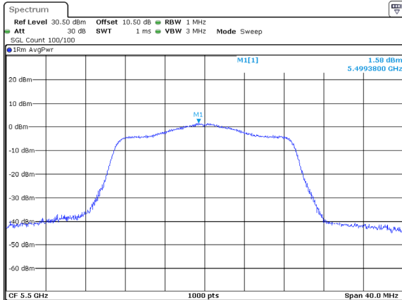
802.11ac20_5500MHz_Chain 2
