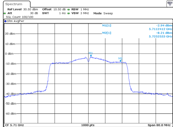
802.11ac40_5710MHz_Chain 1
