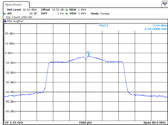
802.11ac40_5550MHz_Chain 2
