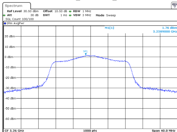
802.11ac20_5260MHz_Chain 1
