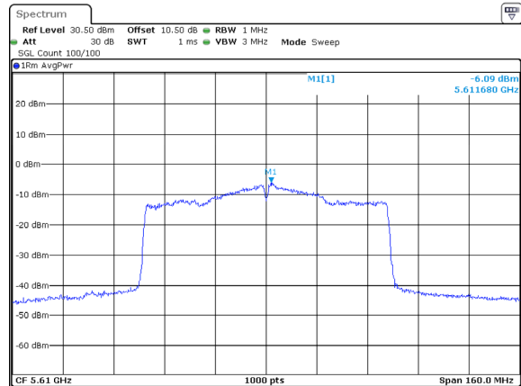
802.11ac80_5610MHz_Chain 1
