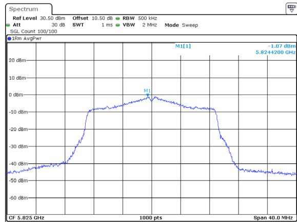
802.11ac20_5825MHz_Chain 2
