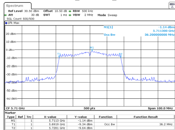
802.11ac40_5710MHz_Chain 1
