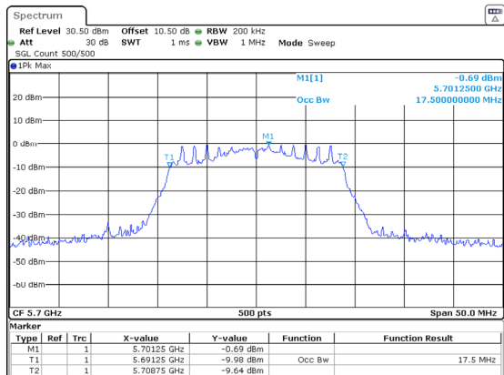
802.11ac20_5700MHz_Chain 1
