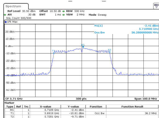
802.11ac40_5710MHz_Chain 2
