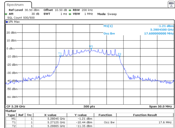
802.11ac20_5280MHz_Chain 1
