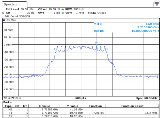
802.11a_5720MHz_Chain 2
