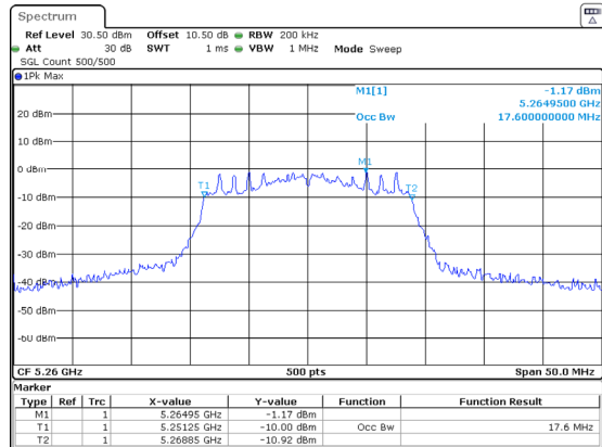
802.11ac20_5260MHz_Chain 1
