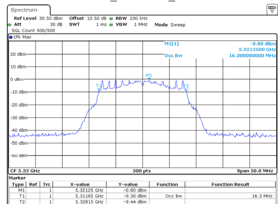
802.11a_5320MHz_Chain 2
