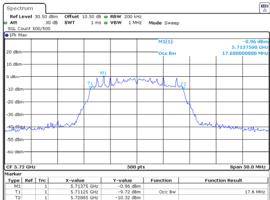
802.11ac20_5720MHz_Chain 1
