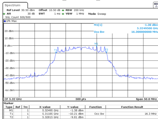
802.11a_5320MHz_Chain 1
