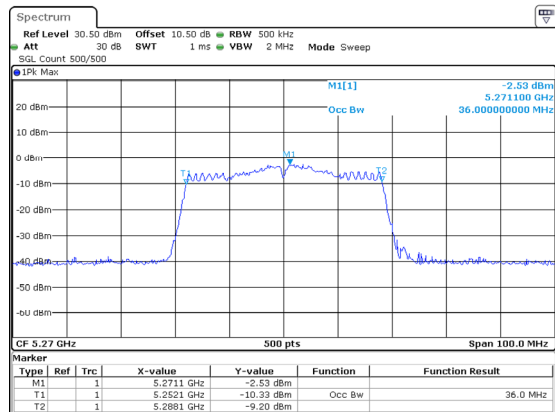
802.11ac40_5270MHz_Chain 2
