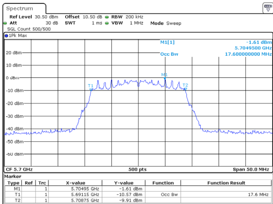
802.11ac20_5700MHz_Chain 2
