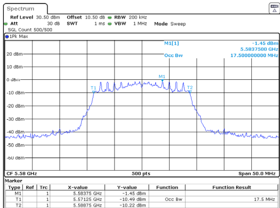
802.11ac20_5580MHz_Chain 1
