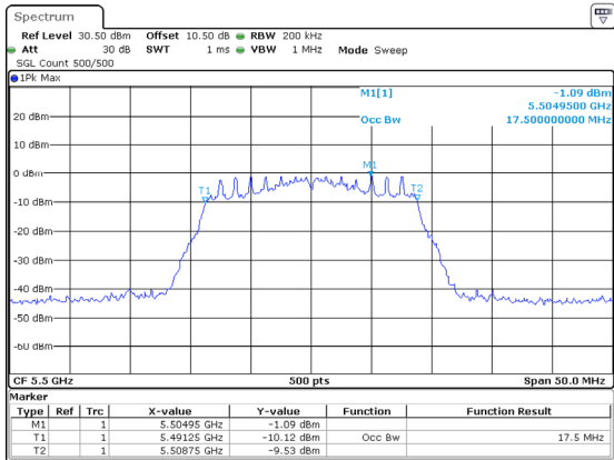
802.11ac20_5500MHz_Chain 2
