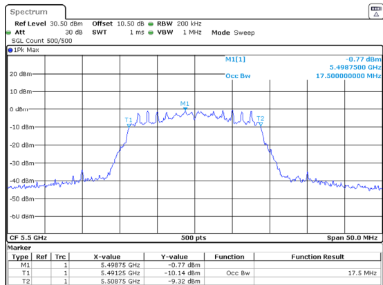
802.11ac20_5500MHz_Chain 1
