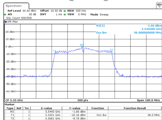
802.11ac40_5550MHz_Chain 2
