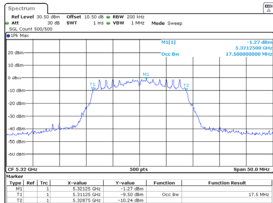
802.11ac20_5320MHz_Chain 1
