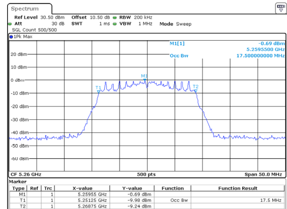
802.11ac20_5260MHz_Chain 2
