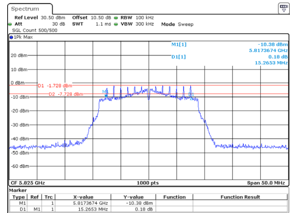
802.11ac20_5825MHz_Chain 2
