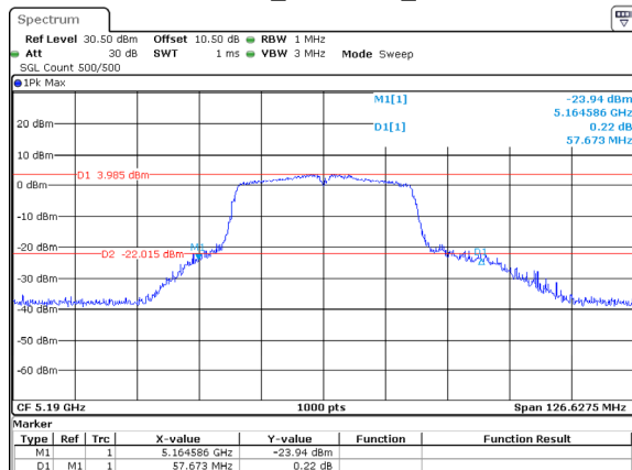
802.11ac40_5190MHz_Chain 2
