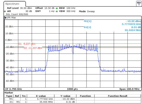
802.11ac40_5795MHz_Chain 2
