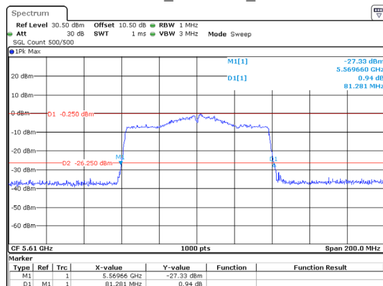
802.11ac80_5610MHz_Chain 2
