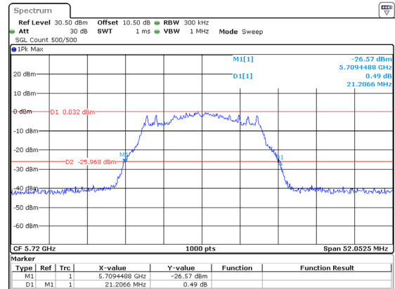
802.11a_5720MHz_Chain 2
