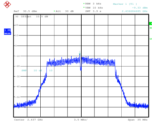
802.11n20_2437MHz_Chain 1
