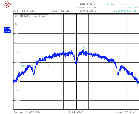
802.11b_2462MHz_Chain 2
