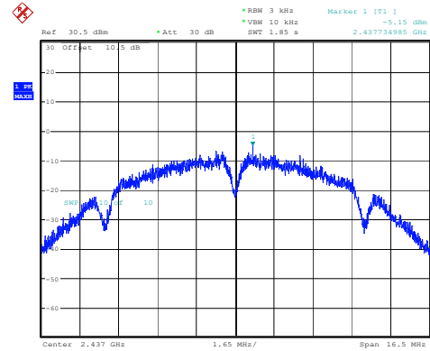
802.11b_2437MHz_Chain 1
