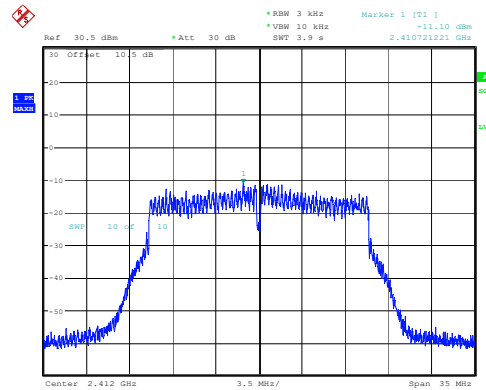
802.11n20_2412MHz_Chain 2
