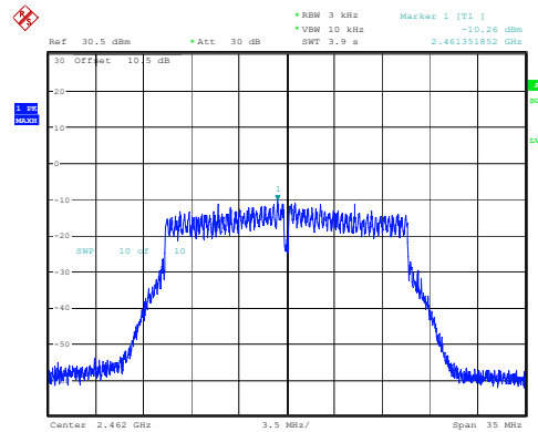
802.11n20_2462MHz_Chain 2
