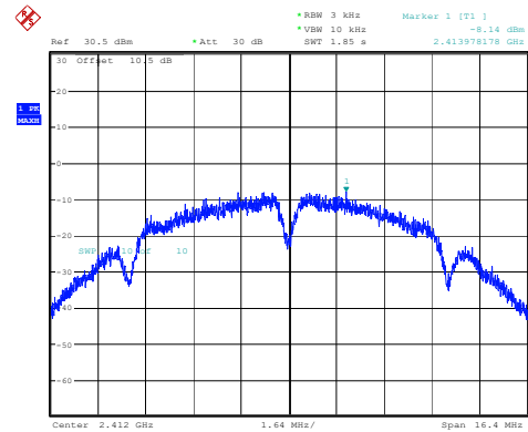
802.11b_2412MHz_Chain 2
