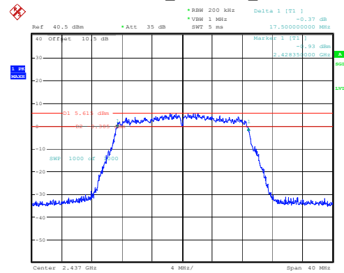
802.11n20_2437MHz_Chain 1
