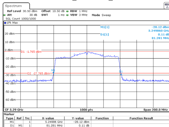
802.11ac80_5290MHz_Chain 1
