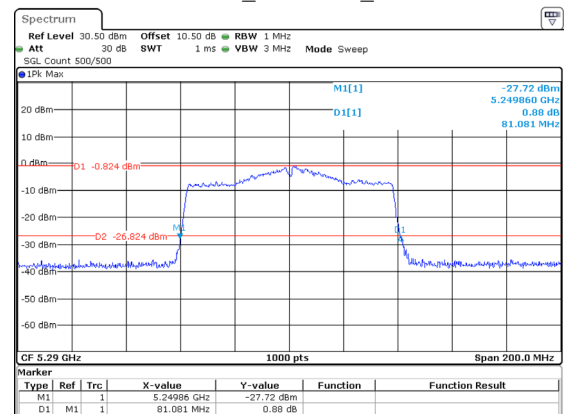
802.11ac80_5290MHz_Chain 2
