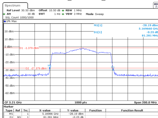
802.11ac80_5210MHz_Chain 1
