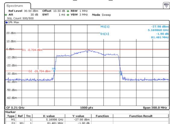
802.11ac80_5210MHz_Chain 2
