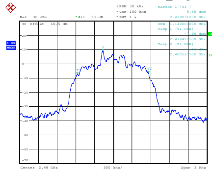
\pi/4 -DQPSK_High
