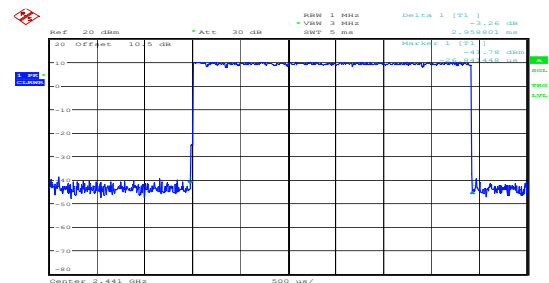
\pi/4 -DQPSK_Hopping_2DH5 2.959ms
