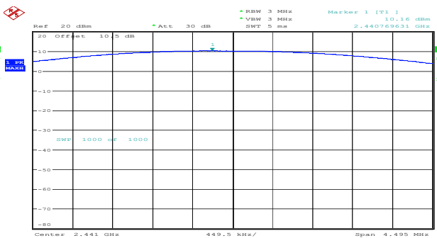
GFSK_Middle 10.16dBm
