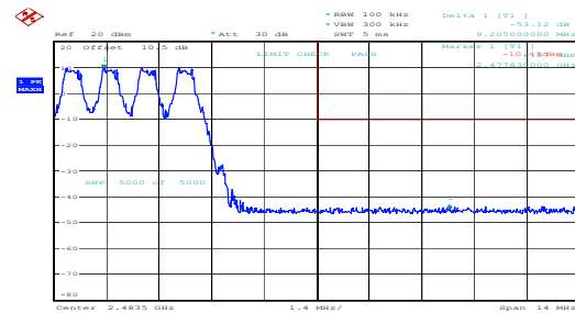
GFSK_Hopping_Upper
