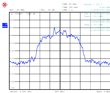
\pi/4 -DQPSK_Middle
