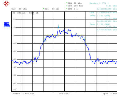
\pi/4 -DQPSK_Low
