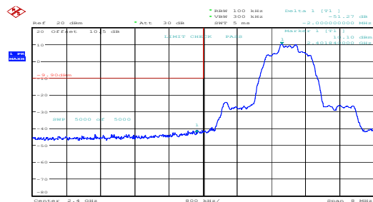
\pi/4 -DQPSK_Low
