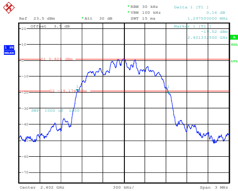
2DH1_Low 1.298MHz
