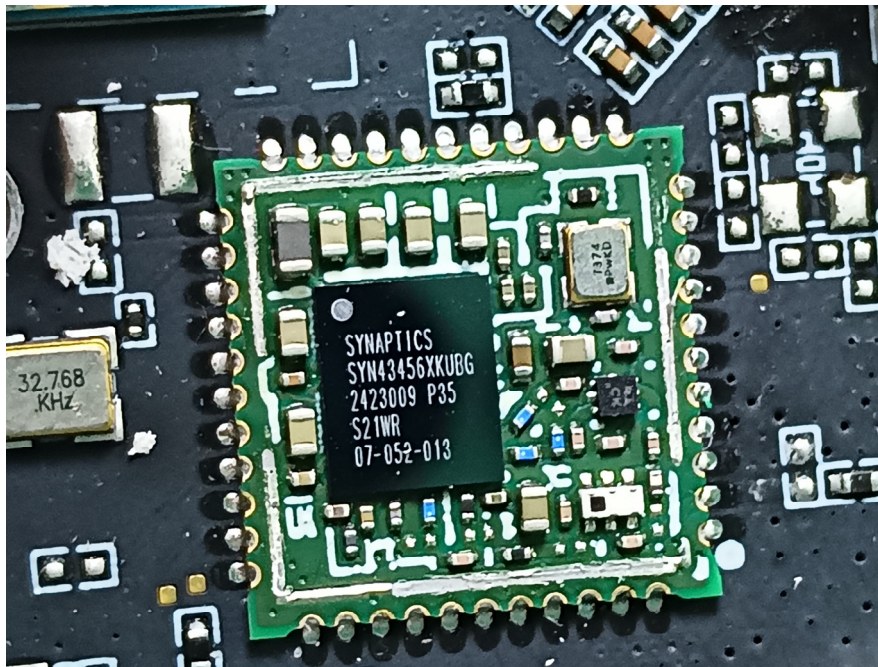
Module YL43456
