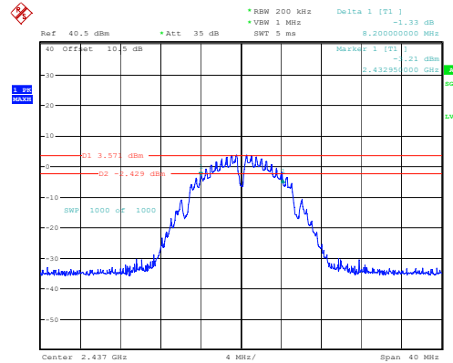
802.11b_2437MHz_Chain 0
