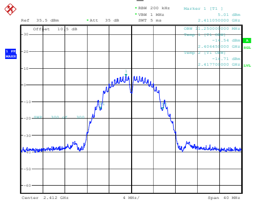
802.11b_2412MHz
