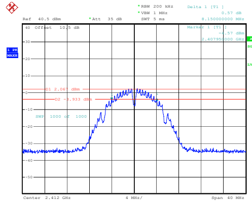
802.11b_2412MHz_Chain 1
