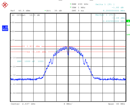
802.11b_2437MHz_Chain 1
