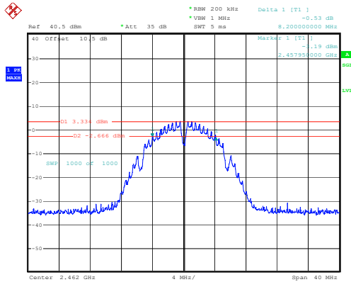
802.11b_2462MHz_Chain 0
