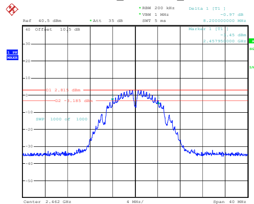
802.11b_2462MHz_Chain 1
