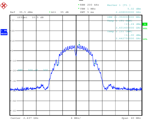
802.11b_2437MHz
