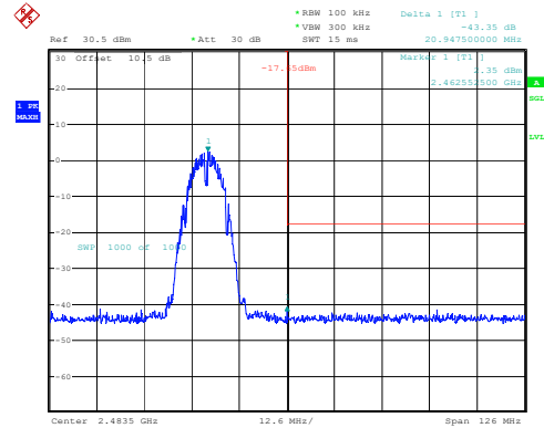
802.11b_2462MHz_Chain 1
