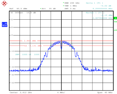
802.11b_2412MHz_Chain 0
