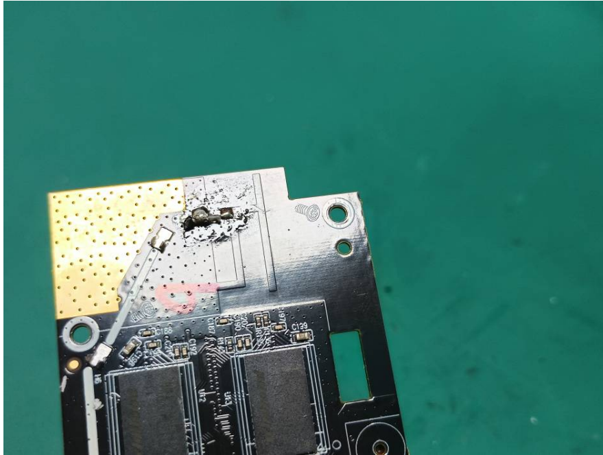
Module YL43752 Wi-Fi ANT2
