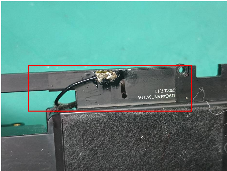
Module YL43456 Wi-Fi ANT
