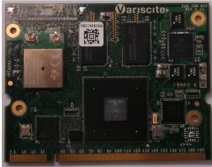
SOM Top with heat sink removed
