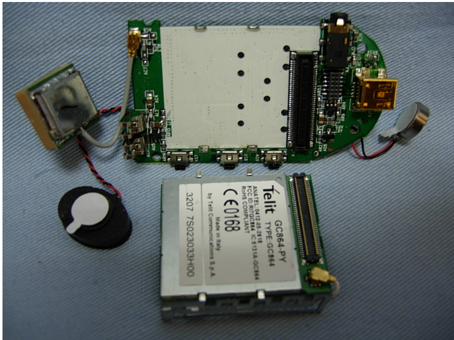
(12) EUT Photo
