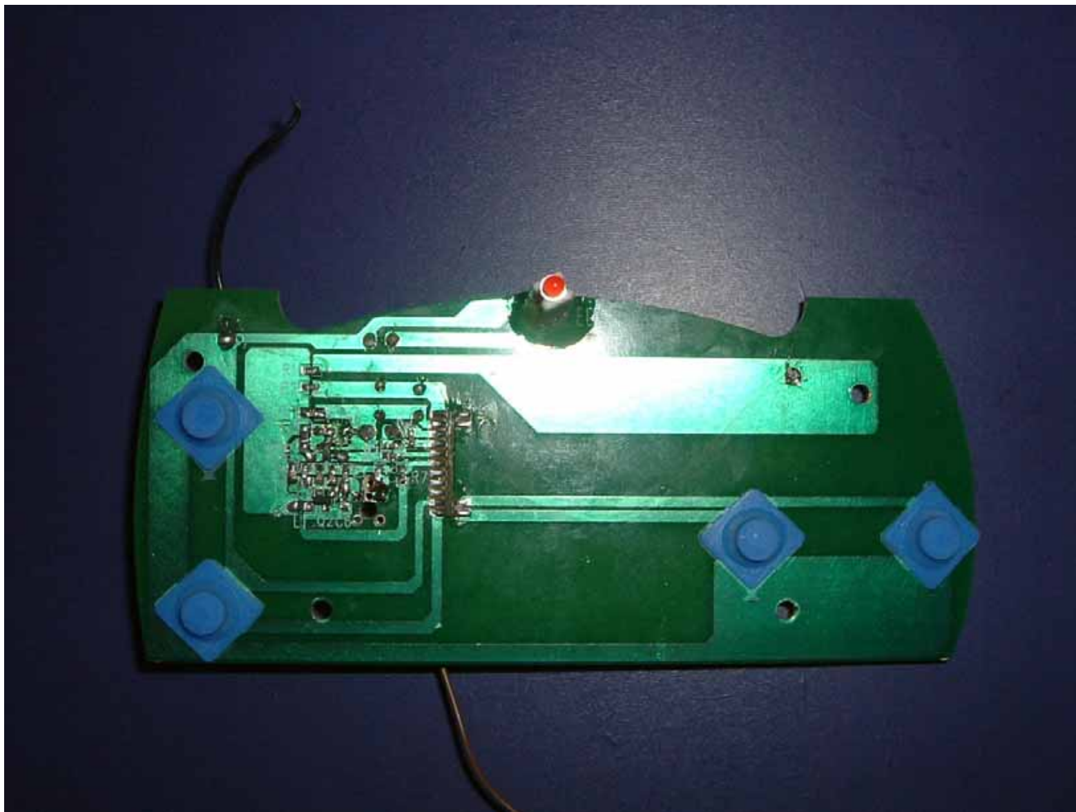
SZ23415T49_PCB2.jpg (1280x960x16M jpeg)
