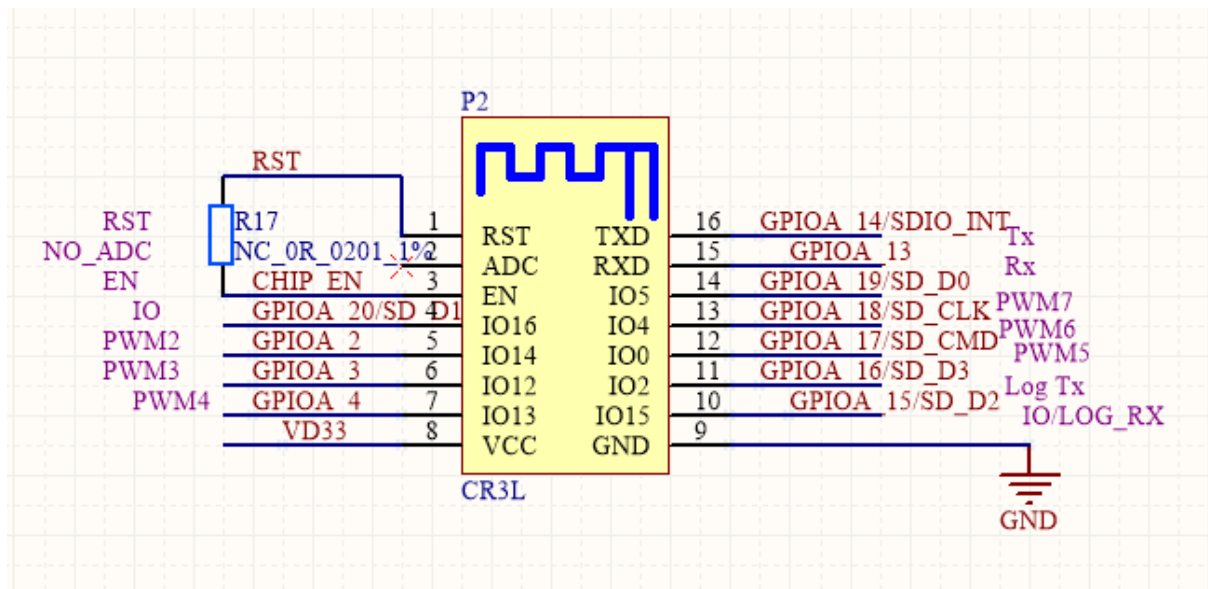
CR3L PCB 封装
