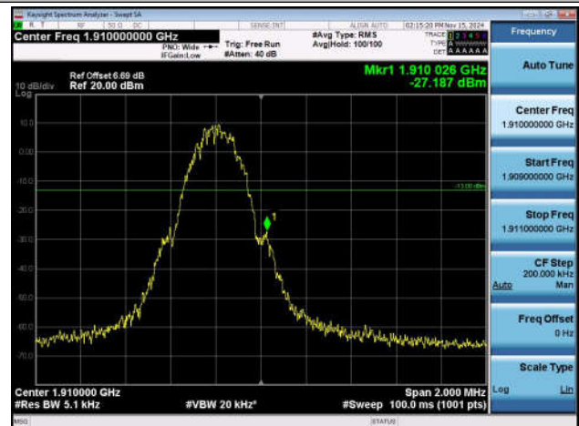
GPRS1900-810-0-PASS
