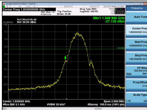
GPRS1900-512-0-PASS
