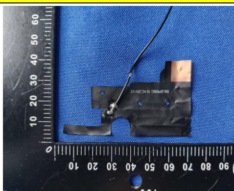
4G DIV ANT (size)
