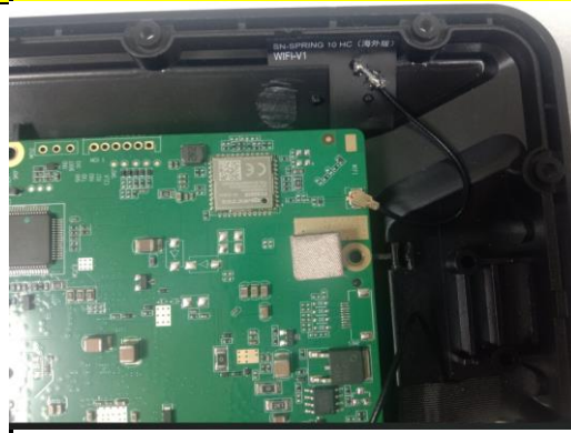
WIFI ANT (Smith+log mag)
