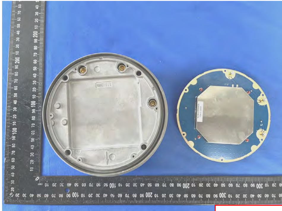
BT/WIFI ANT
