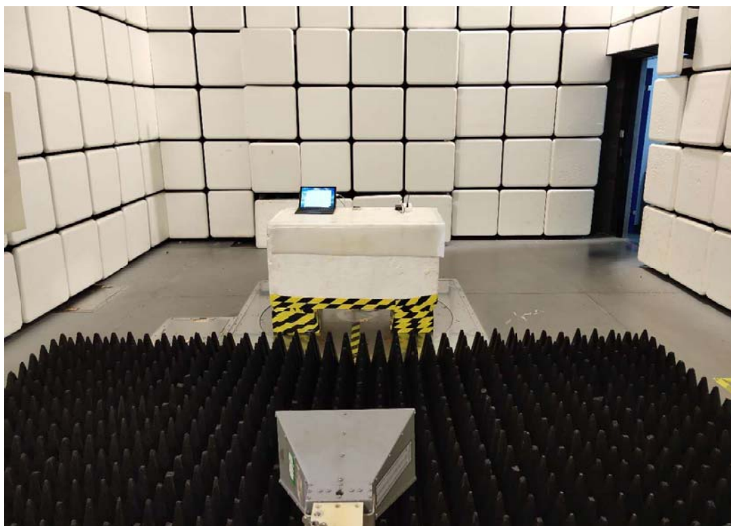
1GHz-18GHz
