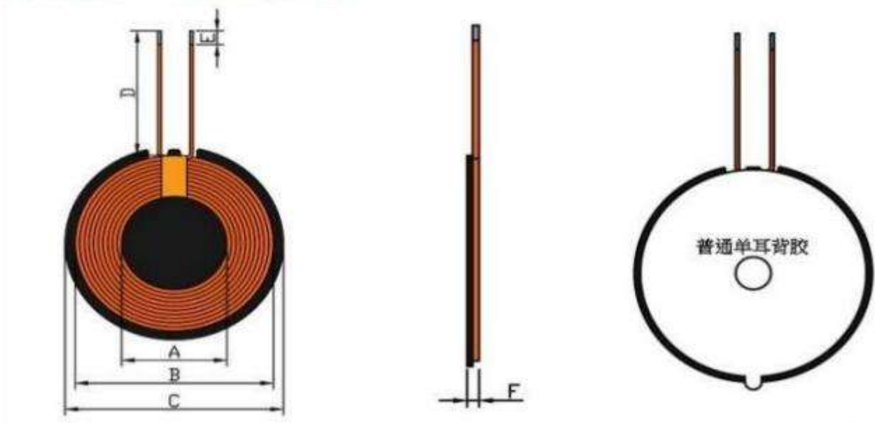
产品尺寸说明 Product Size(单位：MM)
