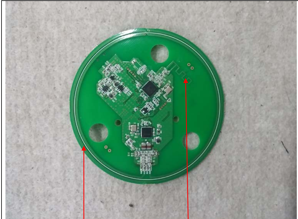
RFID Antenna
