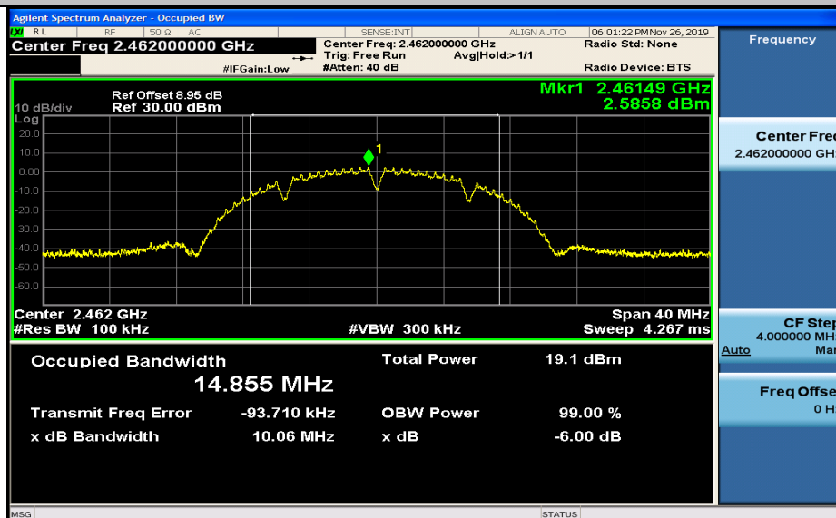
6dB Bandwidth_11B_2462_Ant2
