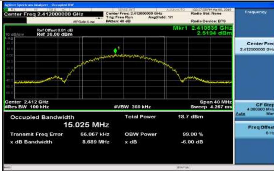
6dB Bandwidth_11B_2412_Ant2
