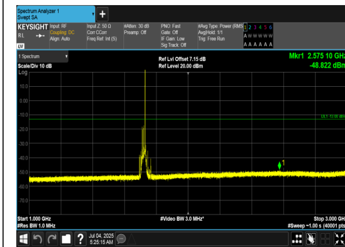
Band66-20MHz-QPSK-132072-1RB#99-1000~3000-PASS
