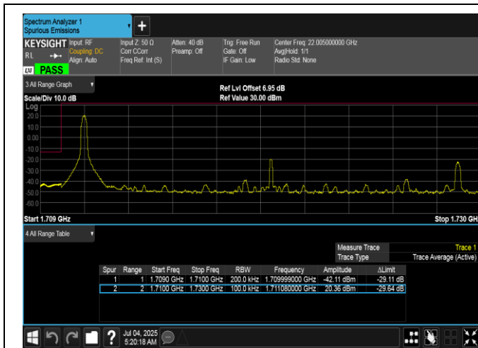
Band66-20MHz-QPSK-132072-1RB#0-PASS
