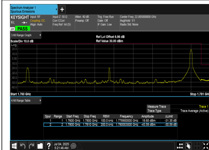
Band66-20MHz-QPSK-132572-1RB#99-PASS
