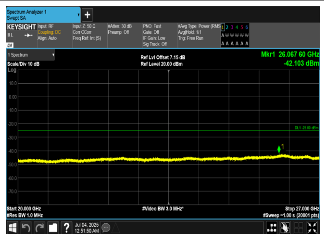
Band7-15MHz-16QAM-20825-1RB#0-20000~27000-PASS
