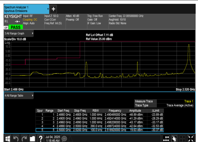
Band7-20MHz-QPSK-20850-1RB#99-PASS
