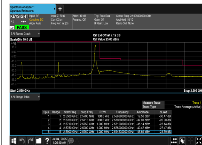
Band7-20MHz-QPSK-21350-1RB#99-PASS
