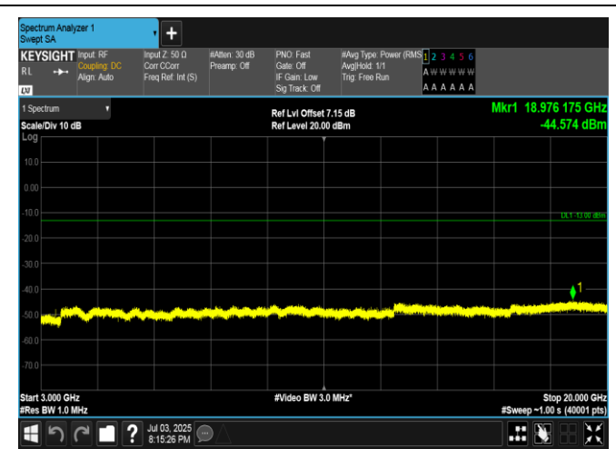
Band4-20MHz-QPSK-20175-1RB#0-3000-20000-PASS
