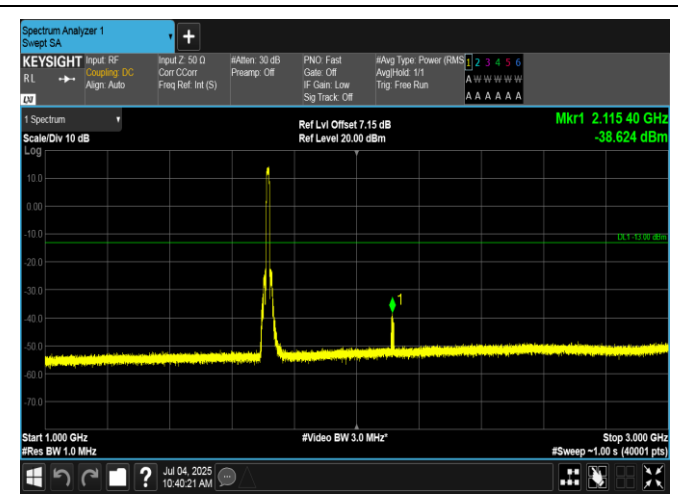
Band4-10MHz-QPSK-20000-50RB#0-1000~3000-PASS
