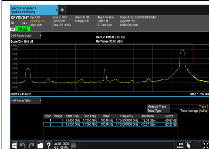
Band4-10MHz-QPSK-20350-1RB#49-PASS
