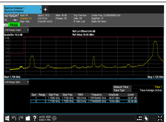
Band4-10MHz-QPSK-20000-1RB#49-PASS
