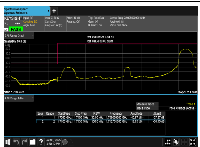
Band4-3MHz-QPSK-19965-1RB#14-PASS
