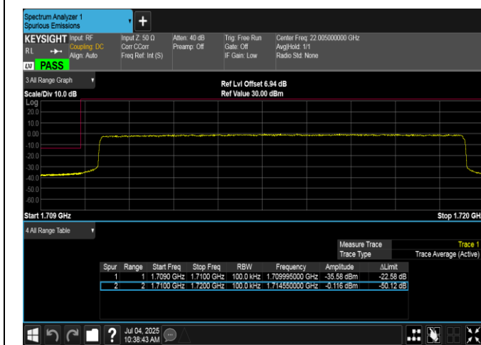
Band4-10MHz-QPSK-20000-50RB#0-PASS
