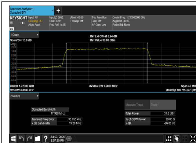
Band4-20MHz-QPSK-20050-100RB#0-PASS
