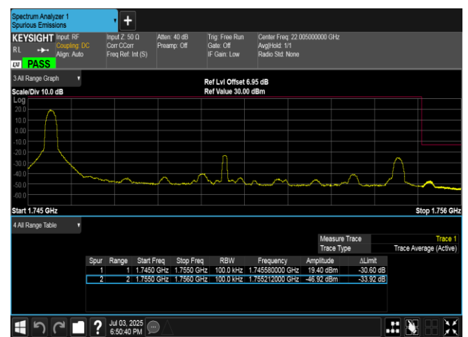
Band4-10MHz-QPSK-20350-1RB#0-PASS
