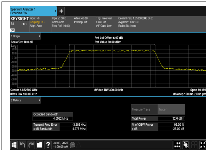
Band2-5MHz-QPSK-18625-25RB#0-PASS
