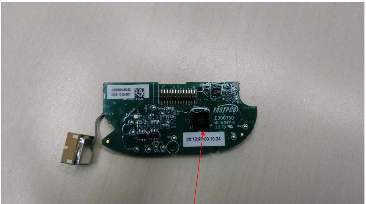
BLE module
