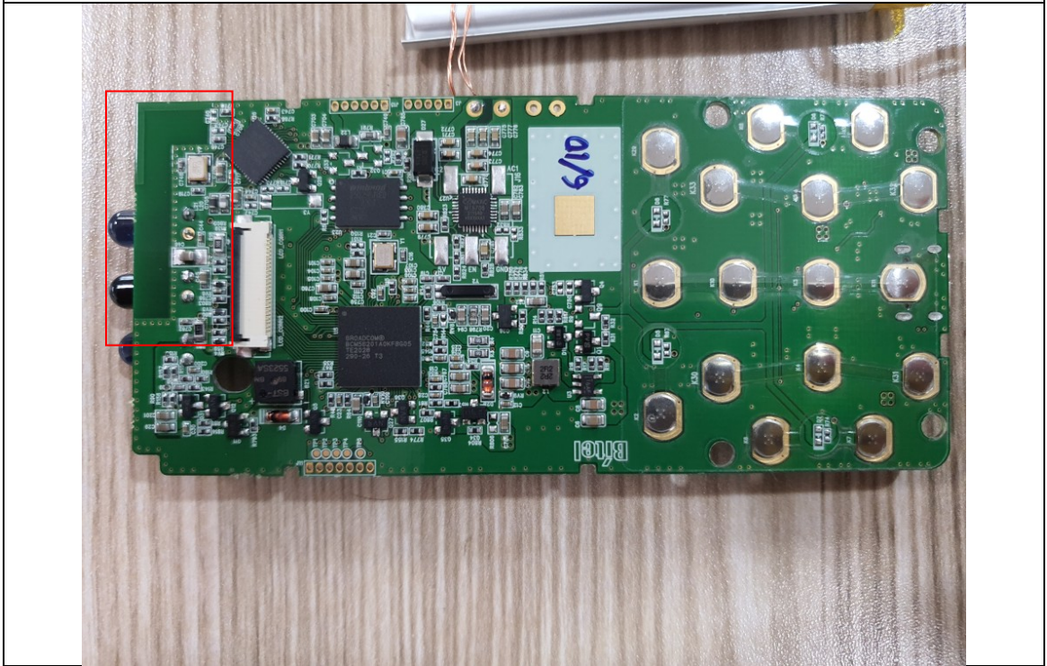
ANTENNA(2.4 GHz)
