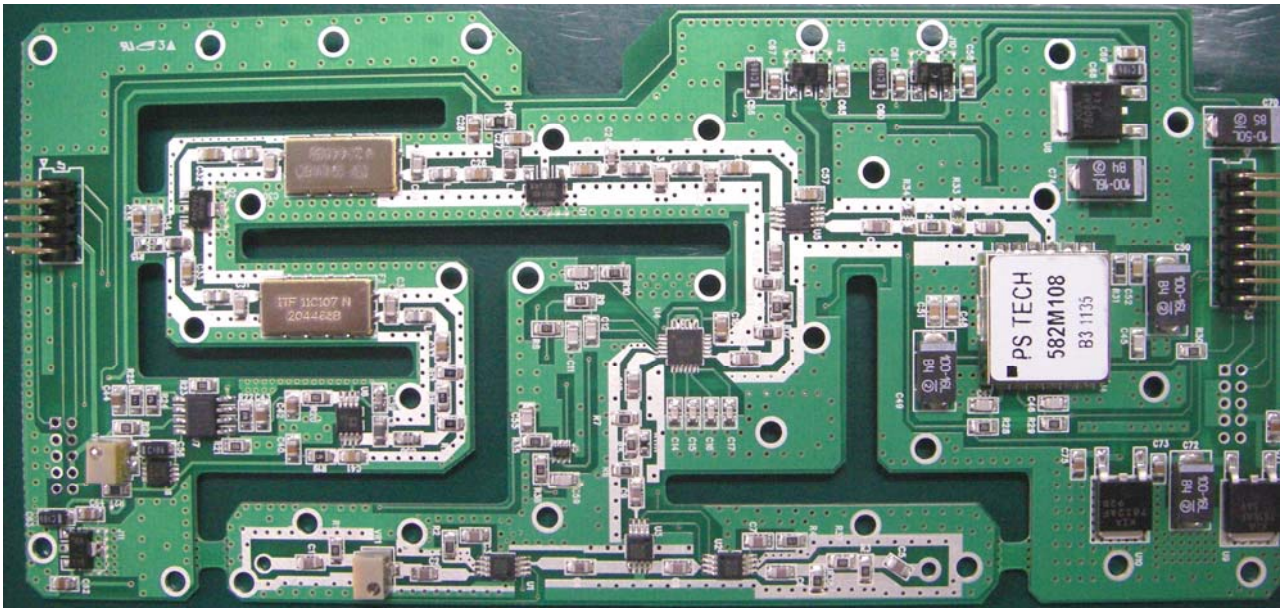
< SA PCB Top View>
