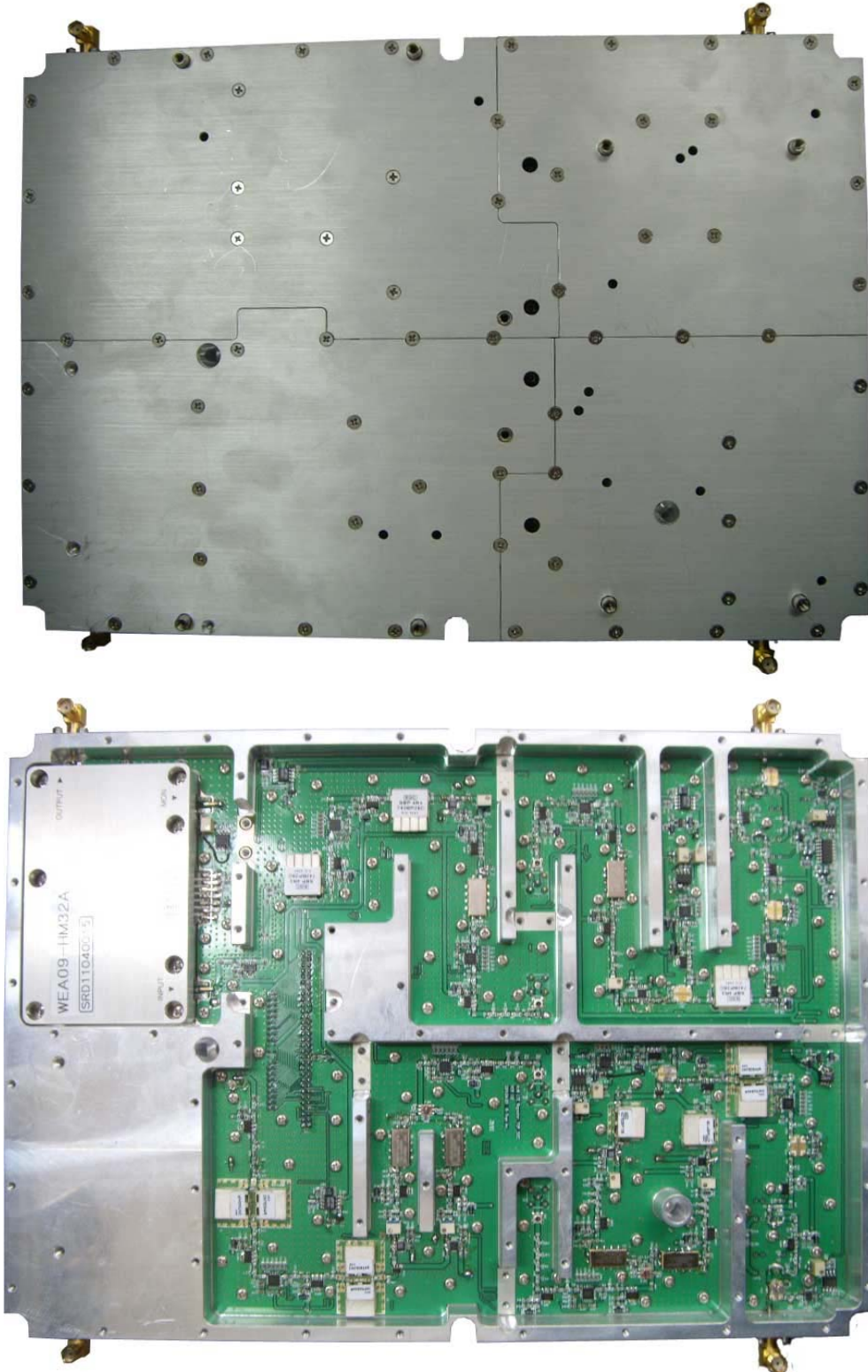
<RFU Top view>
