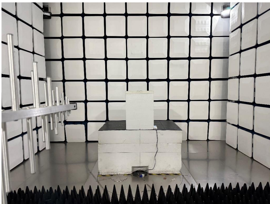
30MHz-1GHz-RFID
